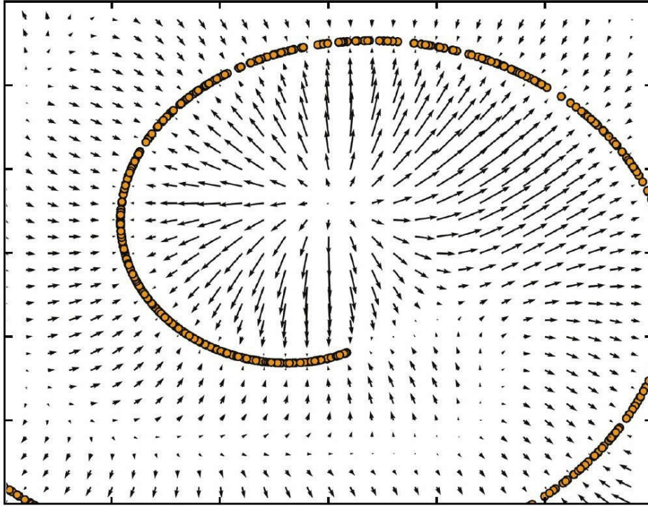
图14.5 由去噪自编码器围绕一维弯曲流形学习的向量场，其中数据集中在二维空间中。每个箭头与重构向量减去自编码器的输入向量后的向量成比例，并且根据隐式估计的概率分布指向较高的概率。向量场在估计的密度函数的最大值处（在数据流形上）和密度函数的最小值处都为零。例如，螺旋臂形成局部最大值彼此连接的一维流形。局部最小值出现在两个臂间隙的中间附近。当重构误差的范数（由箭头的长度示出）很大时，在箭头的方向上移动可以显著增加概率，并且在低概率的地方大多也是如此。自编码器将这些低概率点映射到较高的概率重构。在概率最大的情况下，重构变得更准确，因此箭头会收缩。经Alain and Bengio（2013）许可转载此图
