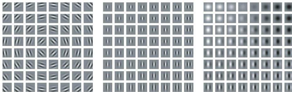
图9.18 具有各种参数设置的Gabor函数。白色表示绝对值大的正权重，黑色表示绝对值大的负权重，背景灰色对应于零权重。（左）控制坐标系的参数具有不同值的Gabor函数，这些参数包括： x_0 、 y_0 和 \tau 。在该网格中的每个Gabor函数被赋予和它在网格中的位置成比例的 x_0 和 y_0 的值，并且 \tau 被选择为使得每个Gabor过滤器对从网格中心辐射出的方向非常敏感。对于其他两幅图， x_0 、 y_0 和 \tau 固定为零。（中）具有不同高斯比例参数 \beta_x 和 \beta_y 的Gabor函数。当我们从左到右通过网格时，Gabor函数被设置为增加宽度（减少 \beta_x ）；当我们从上到下通过网格时，Gabor函数被设置为增加高度（减少 \beta_y ）。对于其他两幅图， \beta 值固定为图像宽度的1.5倍。（右）具有不同的正弦参数 f 和 \phi 的Gabor函数。当我们从上到下移动时， f 增加；当我们从左到右移动时， \phi 增加。对于其他两幅图， \phi 固定为0， f 固定为图像宽度的5倍
