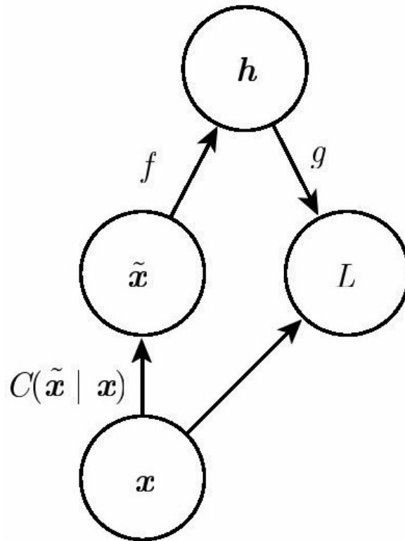
图14.3 去噪自编码器代价函数的计算图。去噪自编码器被训练为从损坏的版本 \tilde{\mathbf{X}} 重构干净数据点 \mathbf{x} 。这可以通过最小化损失 L = -\log p_{\text{decoder}}(\mathbf{x} | \mathbf{h} = f(\tilde{\mathbf{X}})) 实现, 其中 \tilde{\mathbf{X}} 是样本 \mathbf{x} 经损坏过程 C(\tilde{\mathbf{X}} | \mathbf{x}) 后得到的损坏版本。通常, 分布 p_{\text{decoder}} 是因子的分布 (平均参数由前馈网络 g 给出)
