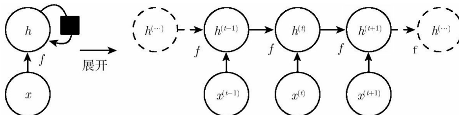
图10.2 没有输出的循环网络。此循环网络只处理来自输入 \mathbf{x} 的信息，将其合并到经过时间向前传播的状态 \mathbf{h} 。（左）回路原理图。黑色方块表示单个时间步的延迟。（右）同一网络被视为展开的计算图，其中每个节点现在与一个特定的时间实例相关联
