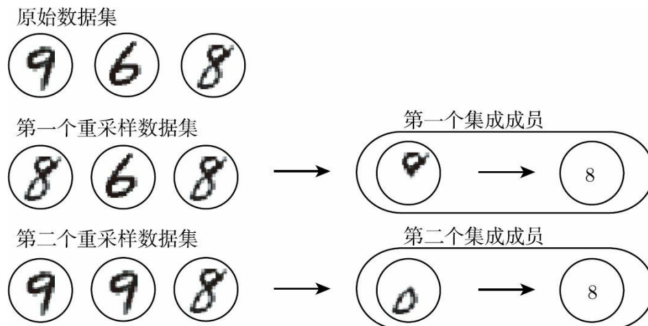
图7.5 描述Bagging如何工作的草图。假设我们在上述数据集（包含一个8、一个6和一个9）上训练数字8的检测器，假设我们制作了两个不同的重采样数据集，Bagging训练程序通过有放回采样构建这些数据集。第一个数据集忽略9并重复8。在这个数据集上，检测器得知数字顶部有
