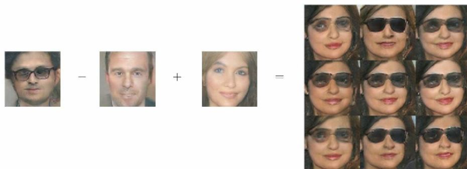
图15.9 生成模型学到了分布式表示，能够从戴眼镜的概念中区分性别概念。如果我们从一个戴眼镜的男人的概念表示向量开始，然后减去一个没戴眼镜的男人的概念表示向量，最后加上一个没戴眼镜的女人的概念表示向量，那么我们会得到一个戴眼镜的女人的概念表示向量。生成模型将所有这些表示向量正确地解码为可被识别为正确类别的图像。图片转载许可自
