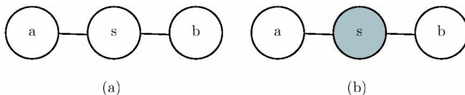
图16.6 (a) 随机变量 a 和随机变量 b 之间穿过 s 的路径是活跃的，因为 s 是观察不到的。这意味着 a 和 b 之间不是分离的。(b) 图中 s 用阴影填充，表示它是可观察的。因为 a 和 b 之间的唯一路径通过 s ，并且这条路径是不活跃的，我们可以得出结论，在给定 s 的条件下 a 和 b 是分离的
