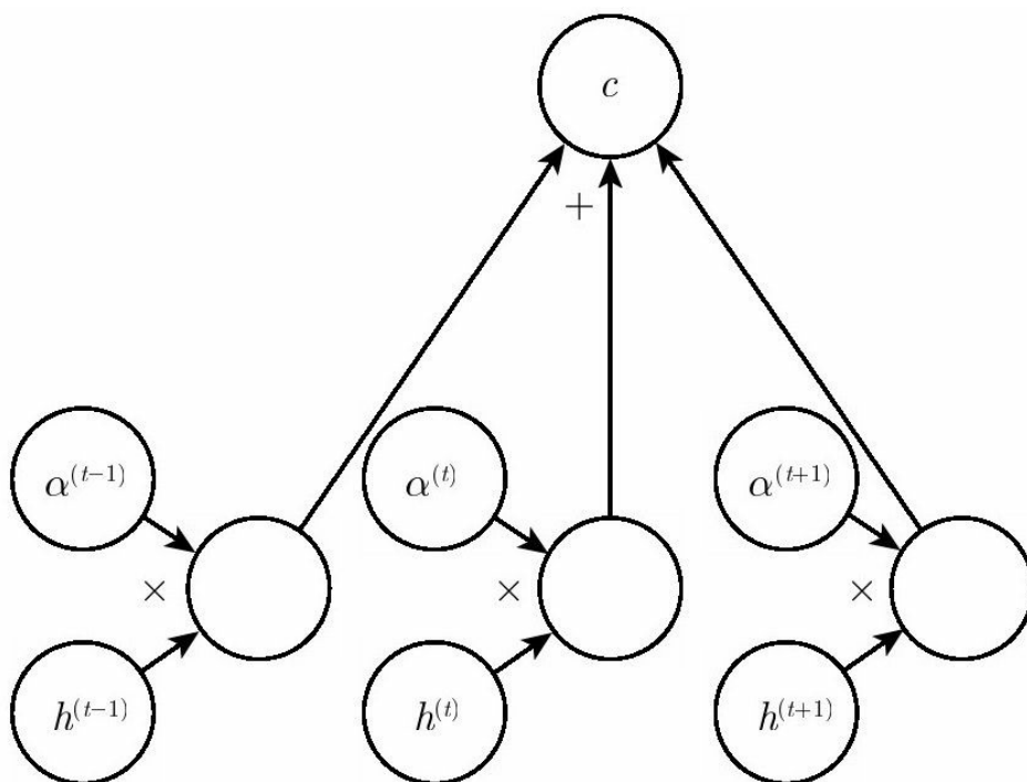
图12.6 由Bahdanau et al. （2015）引入的现代注意力机制，本质上是加权平均。注意力机制对具有权重 \alpha^{(t)} 的特征向量 h^{(t)} 进行加权平均形成上下文向量 c 。在一些应用中，特征向量 h 是
