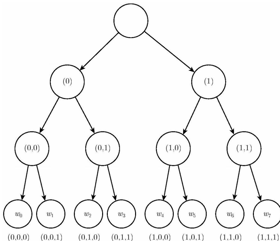
图12.4 词类别简单层次结构的示意图，其中8个词 w_0, \dots, w_7 组织成三级层次结构。树的叶子表示实际特定的词。内部节点表示词的组别。任何节点都可以通过二值决策序列（0=左，1=右）索引，从根到达节点。超类（0）包含类（0,0）和（0,1），其中分别包含词 \{w_0, w_1\} 和 \{w_2, w_3\} 的集合，类似地超类（1）包含类（1,0）和（1,1），分别包含词 \{w_4, w_5\} 和 \{w_6, w_7\} 。如果树充分平衡，则最大深度（二值决策的数量）与词数 |\mathcal{V}| 的对数同阶：从 |\mathcal{V}| 词中选一个词只需执行 \mathcal{O}(\log |\mathcal{V}|) 次操作（从根开始的路径上的每个节点一次操作）。在该示例中，我们乘三次概率就能计算词 y 的概率，这三次概率与从根到节点 y 的路径上每个节点向左或向右的二值决策相关联。令 b_i(y) 为遍历树移向 y 时的第 i 个二值决策。对输出 y 进行采样的概率可以通过条件概率的链式法则分解为条件概率的乘积，其中每个节点由这些位的前缀索引。例如，节点（1,0）对应于前缀 (b_0(w_4)=1, b_1(w_4)=0) ，并且 w_4 的概率可以如下分解：
