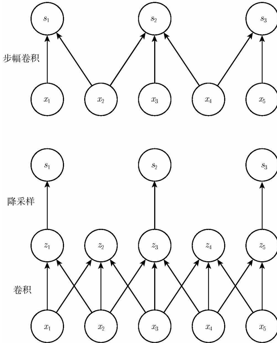
图9.12 带有步幅的卷积。在这个例子中，我们的步幅为2。（上）在单个操作中实现的步幅为2的卷积。（下）步幅大于一个像素的卷积在数学上等价于单位步幅的卷积随后降采样。显然，涉及降采样的两步法在计算上是浪费的，因为它计算了许多将被丢弃的值
