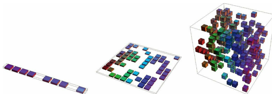
图5.9 当数据的相关维度增大时（从左向右），我们感兴趣的配置数目会随之指数级增长。（左）在这个一维的例子中，我们用一个变量来区分所感兴趣的仅仅10个区域。当每个区域都有足够的样本数时（图中每个样本对应了一个细胞），学习算法能够轻易地泛化得很好。泛化的一个直接方法是估计目标函数在每个区域的值（可能是在相邻区域之间插值）。（中）在二维情况下，对每个变量区分10个不同的值更加困难。我们需要追踪 10 \times 10 = 100 个区域，至少需要很多样本来覆盖所有的区域。（右）三维情况下，区域数量增加到了 10^3 = 1000 ，至少需要那么多的样本。对于需要区分的 d 维以及 v 个值来说，我们需要 O(v^d) 个区域和样本。这就是维数灾难的一个示例。感谢由Nicolas Chapados提供的图片
