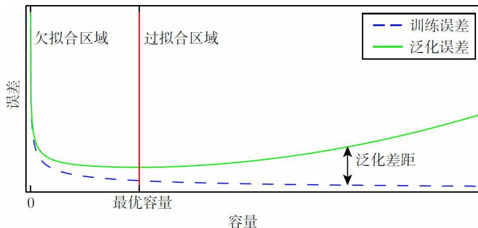
图5.3 容量和误差之间的典型关系。训练误差和测试误差表现得非常不同。在图的左端，训练误差和泛化误差都非常高，这是欠拟合机制（underfitting regime）。当我们增加容量时，训练误差减小，但是训练误差和泛化误差之间的间距却不断扩大。最终，这个间距的大小超过了训
