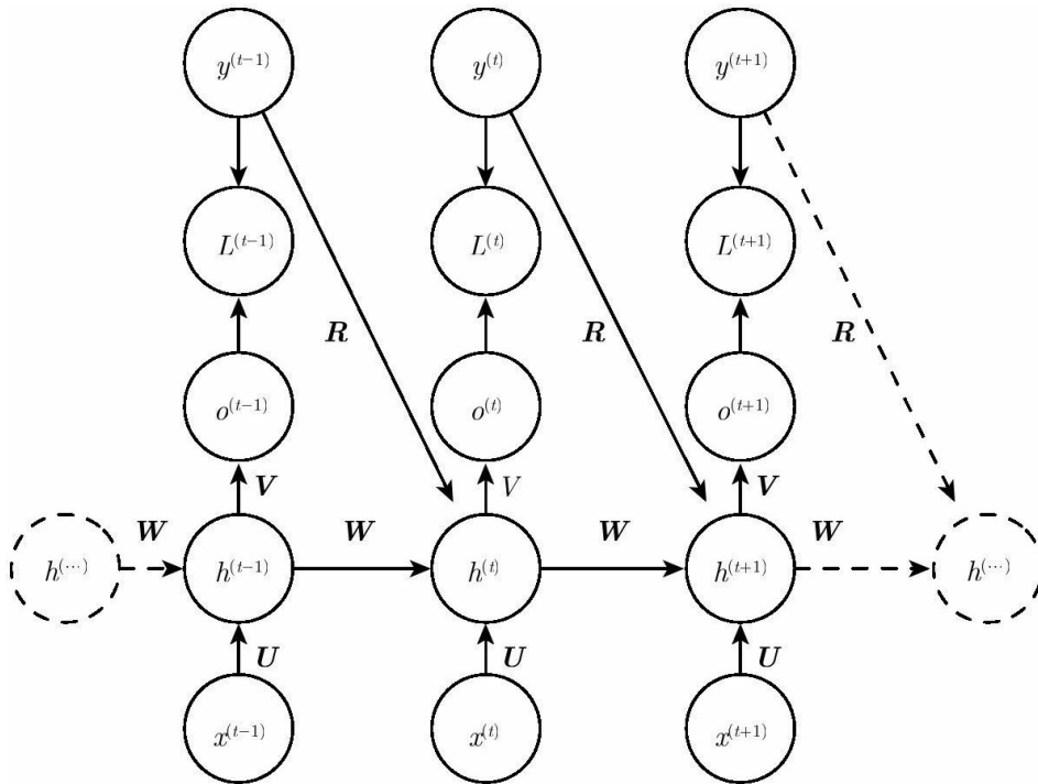
图10.10 将可变长度的 \mathbf{x} 值序列映射到相同长度的 \mathbf{y} 值序列上分布的条件循环神经网络。对比图10.3，此RNN包含从前一个输出到当前状态的连接。这些连接允许此RNN对给定 \mathbf{x} 的序列后相同长度的 \mathbf{y} 序列上的任意分布建模。图10.3的RNN仅能表示在给定 \mathbf{x} 值的情况下， \mathbf{y} 值彼此条件独立的分布
