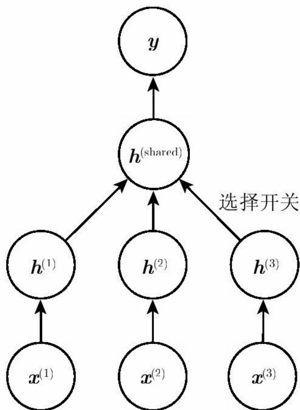
图15.2 多任务学习或者迁移学习的架构示例。输出变量 y 在所有的任务上具有相同的语义，输入变量 x 在每个任务（或者，比如每个用户）上具有不同的意义（甚至可能具有不同的维度）。图上3个任务为 x^{(1)} 、 x^{(2)} 、 x^{(3)} 。底层结构（决定了选择方向）是面向任务的，
