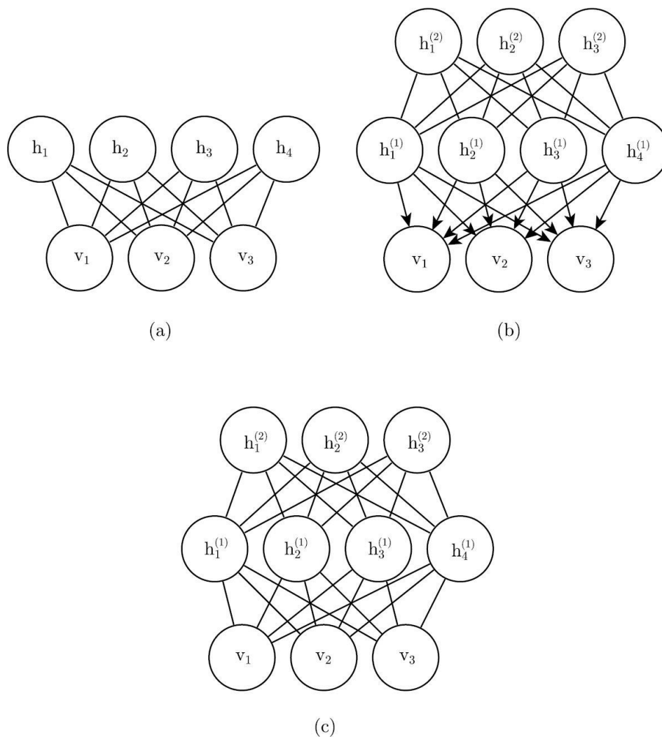
图20.1 可以用受限玻尔兹曼机构建的模型示例。(a)受限玻尔兹曼机本身是基于二分图的无向图模型，图的一部分具有可见单元，另一部分具有隐藏单元。可见单元之间没有连接，隐藏单元之间也没有任何连接。通常每个可见单元连接到每个隐藏单元，但也可以构造稀疏连接的RBM，如卷积RBM。(b)深度信念网络是涉及有向和无向连接的混合图模型。与RBM一样，它也没有层内连接。然而，DBN具有多个隐藏层，因此隐藏单元之间的连接在分开的层中。深度信念网络所需的所有局部条件概率分布都直接复制RBM的局部条件概率分布。或者，我们也可以用完全无向图表示深度信念网络，但是它需要层内连接来捕获父节点间的依赖关系。(c)深度玻尔兹曼机是具有几层潜变量的无向图模型。与RBM和DBN一样，DBM也缺少层内连接。DBM与RBM的联系不如DBN紧密。当从RBM堆栈初始化DBM时，有必要对RBM的参数稍作修改。某些种类的DBM可以直接训练，而不用先训练一组RBM
