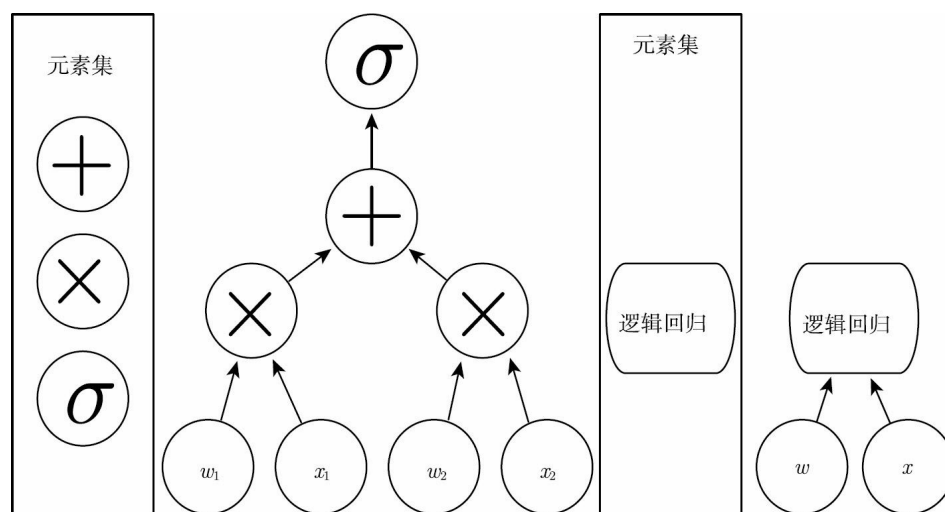
图1.3 将输入映射到输出的计算图表的示意图，其中每个节点执行一个操作。深度是从输入到输出的最长路径的长度，但这取决于可能的计算步骤的定义。这些图中所示的计算是逻辑回归模型的输出， \sigma(w^T x) ，其中 \sigma 是logistic sigmoid函数。如果使用加法、乘法和logistic sigmoid作为计算机语言的元素，那么这个模型深度为3；如果将逻辑回归视为元素本身，那么这个模型深度为1
