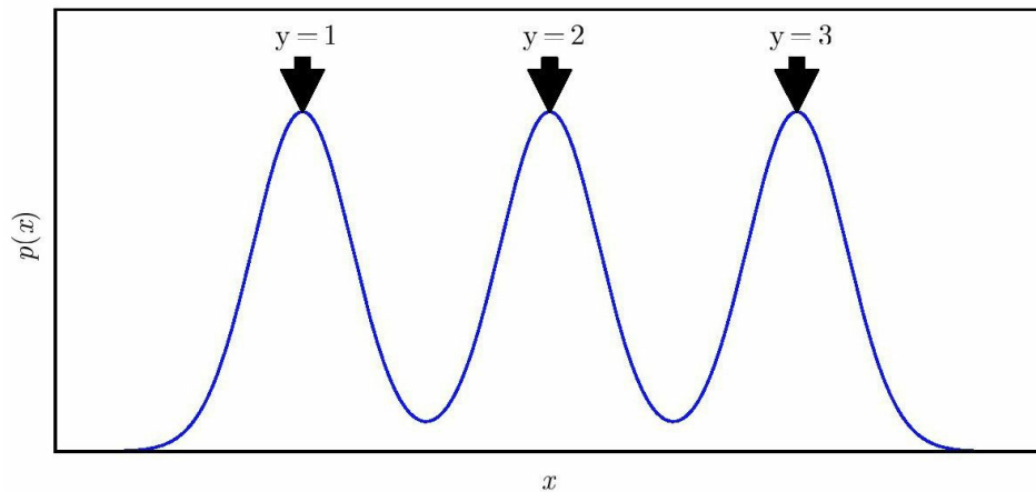
图15.4 混合模型。具有3个混合分量的 \mathbf{x} 上混合密度示例。混合分量的内在本质是潜在解释因子 \mathbf{y} 。因为混合分量（例如，图像数据中的自然对象类别）在统计学上是显著的，所以仅仅使用未标注样本无监督建模 p(\mathbf{x}) 也能揭示解释因子 \mathbf{y}
