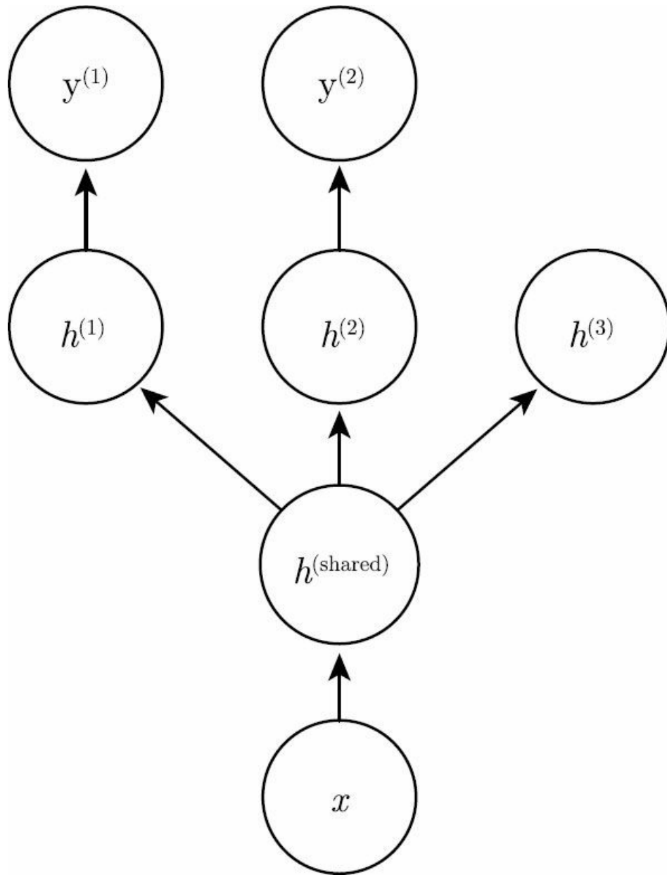
图7.2 多任务学习在深度学习框架中可以以多种方式进行，该图说明了任务共享相同输入但涉及不同目标随机变量的常见情况。深度网络的较低层（无论是监督前馈的，还是包括向下箭头的生成组件）可以跨这样的任务共享，而任务特定的参数（分别与从 h^{(1)} 和 h^{(2)} 进入和发出去的权重）可以在共享表示 h^{(shared)} 之上学习。这里的基本假设是存在解释输入 x 变化的共同因素池，而每个任务与这些因素的子集相关联。在该示例中，额外假设顶层隐藏单元 h^{(1)} 和 h^{(2)} 专用于每个任务（分别预测 y^{(1)} 和 y^{(2)} ），而一些中间层表示 h^{(shared)} 在所有任务之间共享。在无监督学习情况下，一些顶层因素不与输出任务（ h^{(3)} ）的任意一个关联是有意义的：这些因素可以解释一些输入变化但与预测 y^{(1)} 或 y^{(2)} 不相关
