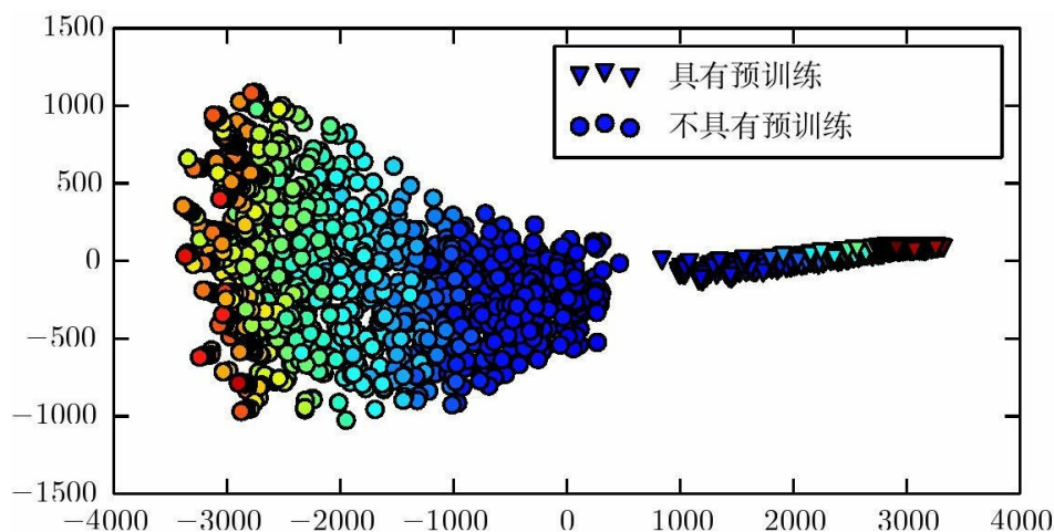
图15.1 在函数空间（并非参数空间，避免从参数向量到函数的多对一映射）不同神经网络学习轨迹的非线性映射的可视化。不同网络采用不同的随机初始化，并且有的使用了无监督预训练，有的没有。每个点对应着训练过程中一个特定时间的神经网络。经Erhan et al. (2010) 许可改编此图。函数空间中的坐标是关于每组输入 \mathbf{x} 和它的一个输出 \mathbf{y} 的无限维向量。Erhan et al. (2010) 将很多特定 \mathbf{x} 的 \mathbf{y} 连接起来，线性投影到高维空间中。然后他们使用
