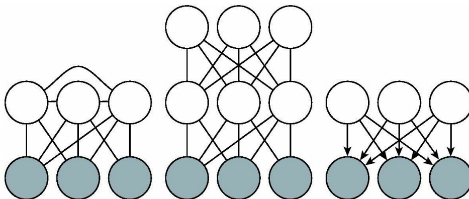
图19.1 深度学习中难以处理的推断问题通常是由于结构化图模型中潜变量的相互作用。这些相互作用产生于一个潜变量与另一个潜变量或者当V-结构的子节点可观察时与更长的激活路径相连。（左）一个隐藏单元存在连接的半受限波尔兹曼机（semi-restricted Boltzmann Machine）（Osindero and Hinton, 2008）。由于存在大量潜变量的团，潜变量的直接连接使得后验分布难以处理。（中）一个深度波尔兹曼机，被分层从而使得不存在层内连接，由于层之间的连接其后验分布仍然难以处理。（右）当可见变量可观察时这个有向模型的潜变量之间存在相互作用，因为每两个潜变量都是共父。即使拥有上图中的某一种结构，一些概率模型依然能够获得易于处理的关于潜变量的后验分布。如果我们选择条件概率分布来引入相对于图结构描述的额外的独立性这种情况也是可能出现的。举个例子，概率PCA的图结构如右图所示，然而由于其条件分布的特殊性质（带有相互正交基向量的线性高斯条件分布）依然能够进行简单的推断
