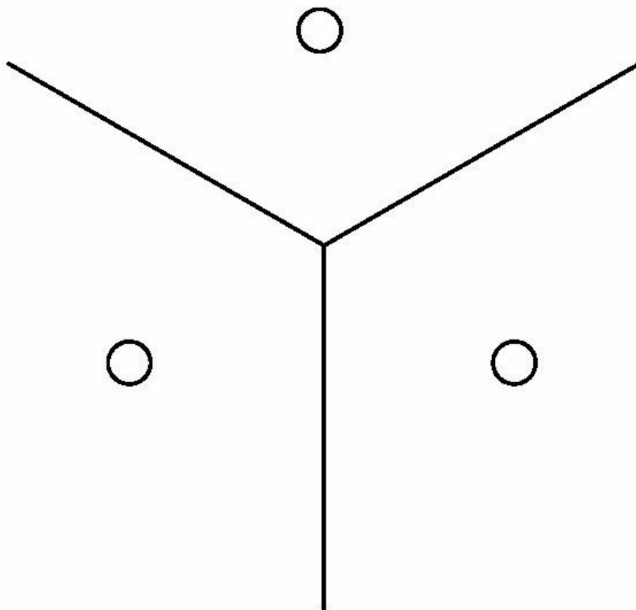
图15.8 最近邻算法如何将输入空间分成不同区域的图示。最近邻算法是一个基于非分布式表示的学习算法的示例。不同的非分布式算法可以具有不同的几何形状，但是它们通常将输入空间分成区域，每个区域具有不同的参数。非分布式方法的优点是，给定足够的参数，它能够拟合一个训练集，而不需要复杂的优化算法。因为它直接为每个区域独立地设置不同的参数。缺点是，非分布式表示的模型只能通过平滑先验来局部地泛化，因此学习波峰波谷多于样本的复杂函数时，该方法是不可行的。和分布式表示的对比，可以参照图15.7
