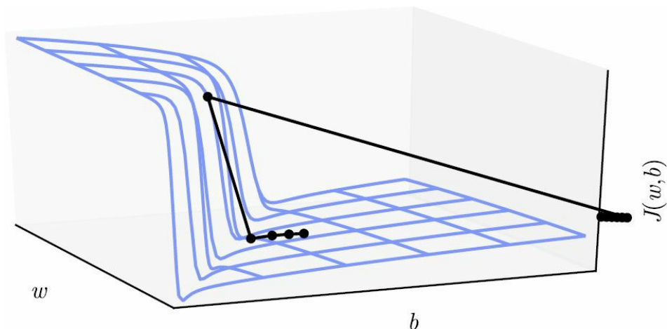
图8.3 高度非线性的深度神经网络或循环神经网络的目标函数通常包含由几个参数连乘而导致的参数空间中尖锐非线性。这些非线性在某些区域会产生非常大的导数。当参数接近这样的悬崖区域时，梯度下降更新可以使参数弹射得非常远，可能会使大量已完成的优化工作成为无功。图经Pascanu et al. (2013a) 许可改编
