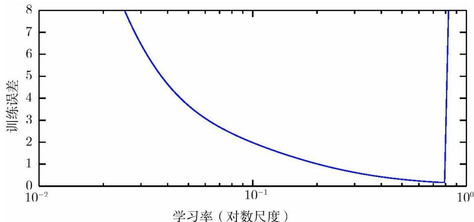
图11.1 训练误差和学习率之间的典型关系。注意，当学习率大于最优值时，误差会有显著的提升。此图针对固定的训练时间，越小的学习率有时候可以以一个正比于学习率减小量的因素来减慢训练过程。泛化误差也会得到类似的曲线，由于正则项作用在学习率过大或过小处比较复杂。一个糟糕的优化从某种程度上说可以避免过拟合，即使是训练误差相同的点也会拥有完全不同的泛化误差
