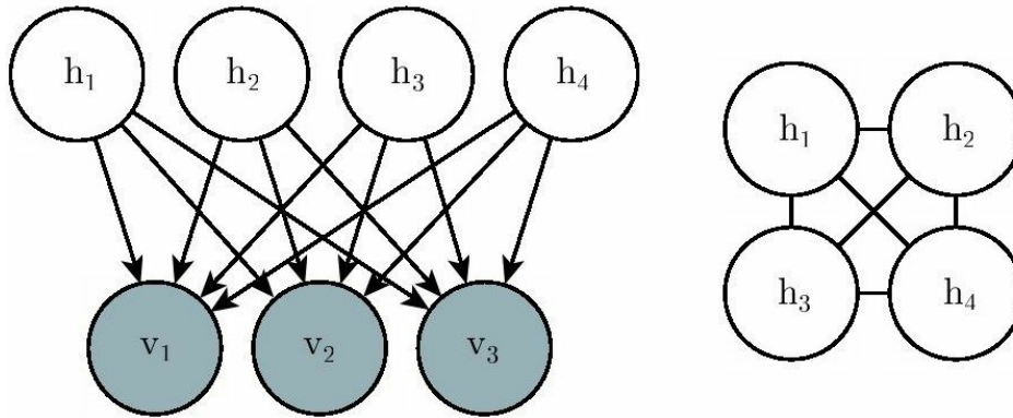
图19.2 包含4个隐藏单元的二值稀疏编码的图结构。（左） p(\mathbf{h}, \mathbf{v}) 的图结构。要注意边是有向的，每两个隐藏单元都是每个可见单元的共父。（右） p(\mathbf{h}, \mathbf{v}) 的图结构。为了解释共父之间的活跃路径，后验分布所有隐藏单元之间都有边
