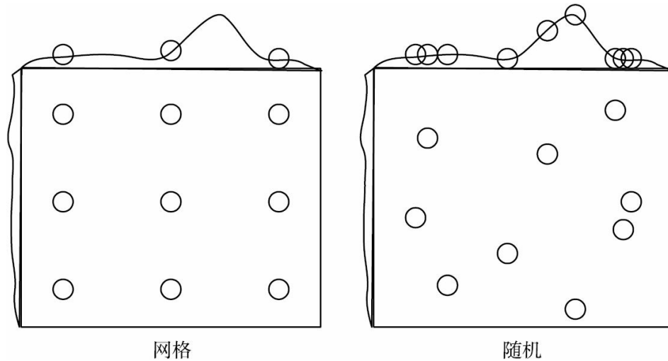
图11.2 网格搜索和随机搜索的比较。为了便于说明，我们只展示两个超参数的例子，但是我们关注的问题中超参数个数通常会更多。（左）为了实现网格搜索，我们为每个超参数提供了一个值的集合。搜索算法对每一种在这些集合的交叉积中的超参数组合进行训练。（右）为了实现随机搜索，我们给联合超参数赋予了一个概率分布。通常超参数之间是相互独立的。常见的这种分布的选择是均匀分布或者是对数均匀（从对数均匀分布中抽样，就是对从均匀分布中抽取的样本进行指数运算）的。然后这些搜索算法从联合的超参数空间中采样，然后运行每一个样本。网格搜索和随机搜索都运行了验证集上的误差并返回了最优的解。这个图说明了通常只有一个超参数对结果有着重要的影响。在这个例子中，只有水平轴上的超参数对结果有重要的作用。网格搜索将大量的计算浪费在指数量级的对结果无影响的超参数中，相比之下随机搜索几乎每次测试都测试了对结果有影响的每个超参数的独一无二的值。此图经Bergstra and Bengio (2011) 允许转载
