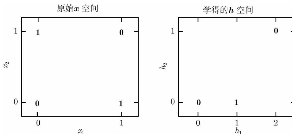
图6.1 通过学习一个表示来解决XOR问题。图上的粗体数字标明了学得的函数必须在每个点输出的值。（左）直接应用于原始输入的线性模型不能实现XOR函数。当 x_1 = 0 时，模型的输出必须随着 x_2 的增大而增大。当 x_1 = 1 时，模型的输出必须随着 x_2 的增大而减小。线性模型必须对 x_2 使用固定的系数 w_2 。因此，线性模型不能使用 x_1 的值来改变 x_2 的系数，从而不能解决这个问题。（右）在由神经网络提取的特征表示的变换空间中，线性模型现在可以解决这个问题了。在我们的示例解决方案中，输出必须为1的两个点折叠到了特征空间中的单个点。换句话说，非线性特征将 \mathbf{x} = [1, 0]^T 和 \mathbf{x} = [0, 1]^T 都映射到了特征空间中的单个点
