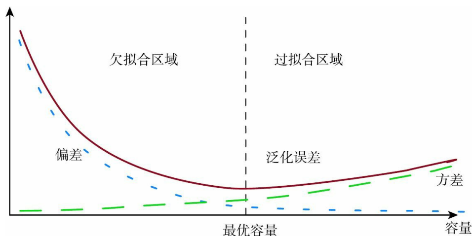
图5.6 当容量增大（x轴）时，偏差（用点表示）随之减小，而方差（虚线）随之增大，使得泛化误差（加粗曲线）产生了另一种U形。如果我们沿着轴改变容量，会发现最佳容量，当容量小于最佳容量会呈现欠拟合，大于时导致过拟合。这种关系与第5.2节以及图5.3中讨论的容量、欠拟合和过拟合之间的关系类似
