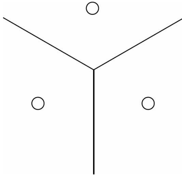
图5.10 最近邻算法如何划分输入空间的示例。每个区域内的一个样本（这里用圆圈表示）定义了区域边界（这里用线表示）。每个样本相关的 y 值定义了对应区域内所有数据点的输出。由最近邻定义并且匹配几何模式的区域被称为Voronoi图。这些连续区域的数量不会比训练样本的数量增加得更快。尽管此图具体说明了最近邻算法的效果，其他的单纯依赖局部光滑先验的机器学习算法也表现出了类似的泛化能力：每个训练样本仅仅能告诉学习者如何在其周围的相邻区域泛化
