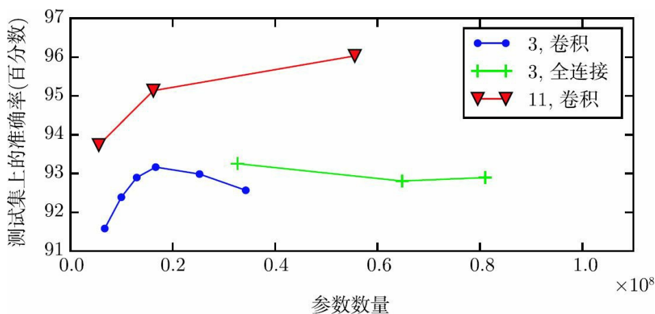
图6.7 参数数量的影响。更深的模型往往表现更好。这不仅仅是因为模型更大。Goodfellow et al. (2014d) 的实验表明，增加卷积网络层中参数的数量，但是不增加它们的深度，在提
