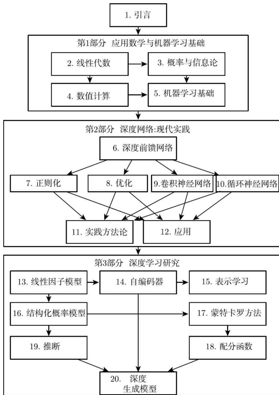
图1.6 本书的高层组织结构的流程图。从一章到另一章的箭头表示前一章是理解后一章的必备内容
