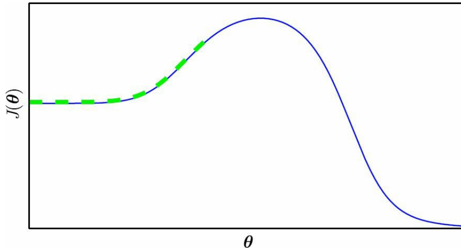
图8.4 如果局部表面没有指向全局解，基于局部下坡移动的优化可能就会失败。这里我们提供一个例子，说明即使在没有鞍点或局部极小值的情况下，优化过程会如何失败。此例中的代价函数仅包含朝向低值而不是极小值的渐近线。在这种情况下，造成这种困难的主要原因是初始化在“山”的错误一侧，并且无法遍历。在高维空间中，学习算法通常可以环绕过这样的高山，但是相关的轨迹可能会很长，并且导致过长的训练时间，如图8.2所示
