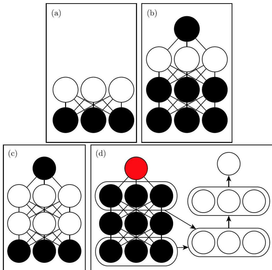
图20.4 用于分类MNIST数据集的深度玻尔兹曼机训练过程 (Salakhutdinov and Hinton, 2009a; Srivastava et al. , 2014)。(a) 使用CD近似最大化 \log P(\mathbf{v}) 来训练RBM。(b) 训练第二个RBM，使用CD-k近似最大化 \log P(\mathbf{h}^{(1)} | y) 来建模 \mathbf{h}^{(1)} 和目标类 y ，其中 \mathbf{h}^{(1)} 采自第一个RBM条件于数据的后验。在学习期间将 k 从1增加到20。(c) 将两个RBM组合为DBM。使用 k=5 的随机最大似然训练，近似最大化 \log P(\mathbf{v}, y) 。(d) 将 y 从模型中删除。定义新的一组特征 \mathbf{h}^{(1)} 和 \mathbf{h}^{(2)} ，可在缺少 y 的模型中运行均匀场推断后获得。使用这些特征作为MLP的输入，其结构与均匀场的额外轮相同，并且具有用于估计 y 的额外输出层。初始化MLP的权重与DBM的权重相同。使用随机梯度下降和Dropout训练MLP近似最大化 \log P(y | \mathbf{v}) 。图来自Goodfellow et al (2013d)
