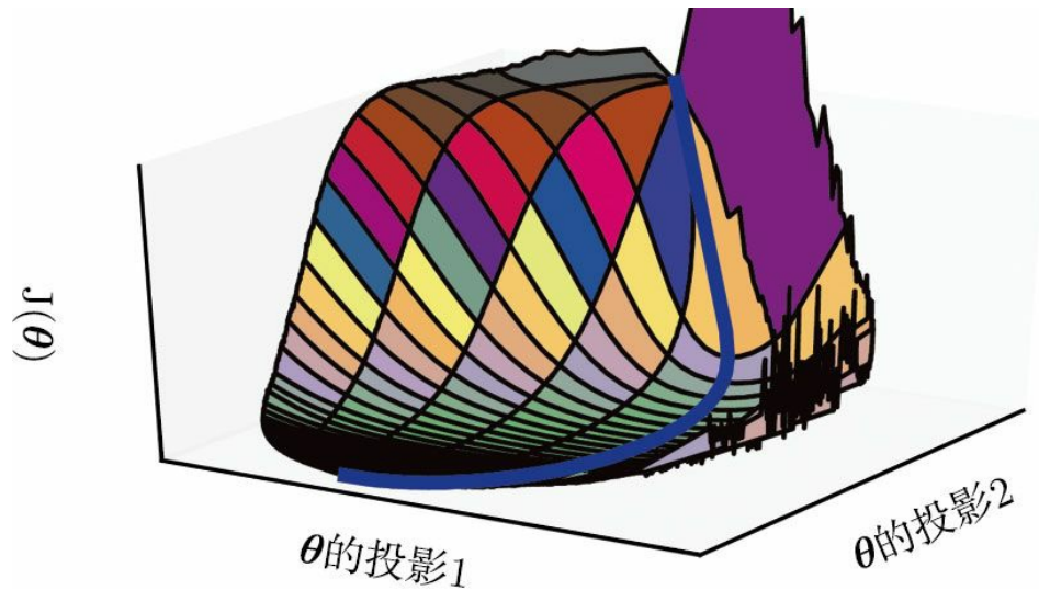
图8.2 神经网络代价函数的可视化。这些可视化对应用于真实对象识别和自然语言处理任务的前馈神经网络、卷积网络和循环网络而言是类似的。令人惊讶的是，这些可视化通常不会显示出很多明显的障碍。大约2012年，在随机梯度下降开始成功训练非常大的模型之前，相比这些投影所显示的神经网络代价函数的表面通常被认为有更多的非凸结构。该投影所显示的主要障碍是初始参数附近的高代价鞍点，但如由蓝色路径所示，SGD训练轨迹能轻易地逃脱该鞍点。大多数训练时间花费在横穿代价函数中相对平坦的峡谷，可能由于梯度中的高噪声，或该区域中Hessian矩阵的病态条件，或者需要经过间接的弧路径绕过图中可见的高“山”。图经
