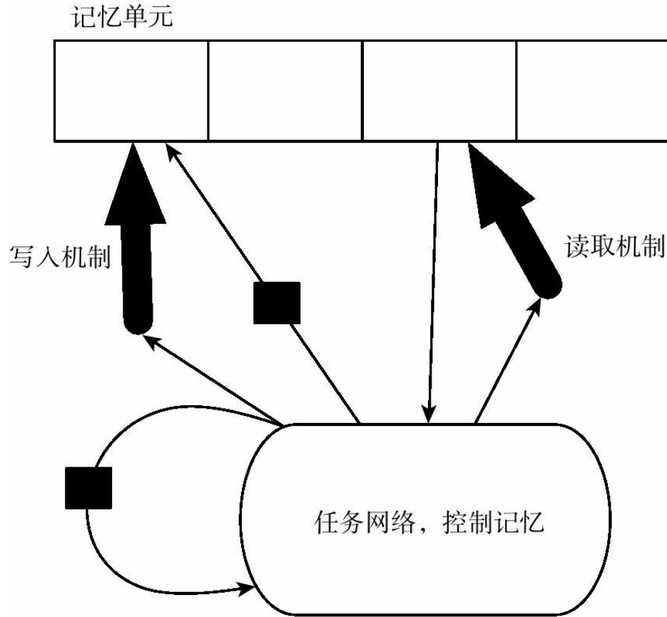
图10.18 具有外显记忆网络的示意图，具备神经网络图灵机的一些关键设计元素。在此图中，我们将模型的“表示”部分（“任务网络”，这里是底部的循环网络）与存储事实的模型（记忆单元的集合）的“存储器”部分区分开。任务网络学习“控制”存储器，决定从哪里读取以及在哪里写入（通过读取和写入机制，由指向读取和写入地址的粗箭头指示）
