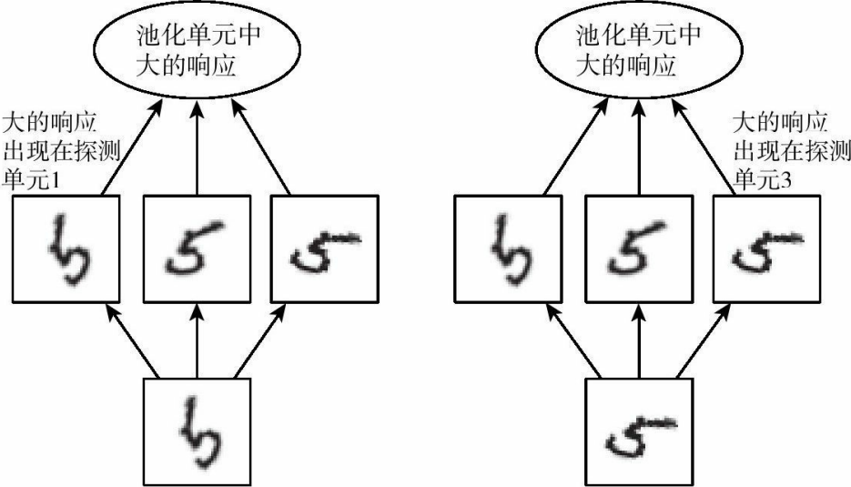
图9.9 学习不变性的示例。使用分离的参数学得多个特征，再使用池化单元进行池化，可以学得对输入的某些变换的不变性。这里我们展示了用三个学得的过滤器和一个最大池化单元可以学得对旋转变换的不变性。这三个过滤器都旨在检测手写的数字5。每个过滤器尝试匹配稍微不同方向的5。当输入中出现5时，相应的过滤器会匹配它并且在探测单元中引起大的激活。然后，无论哪个探测单元被激活，最大池化单元都具有大的激活。我们在这里演示了网络如何处理两个不同的输入，这导致两个不同的探测单元被激活，然而对池化单元的影响大致相同。这个原则在maxout网络（Goodfellow et al. ，2013b）和其他卷积网络中更有影响。空间位置上的最大池化对于平移是天然不变的。这种多通道方法只在学习其他变换时是必要的
