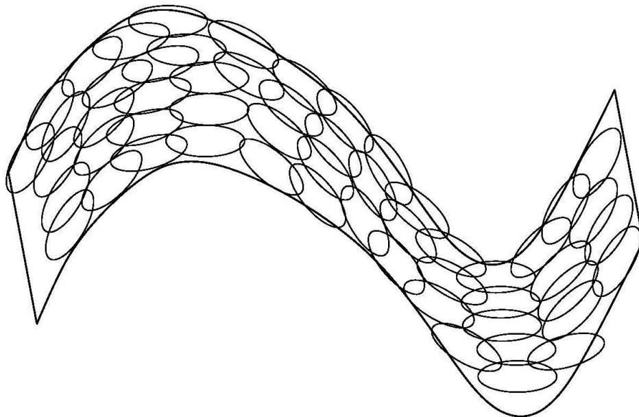
图14.9 如果每个位置处的切平面（见图14.6）是已知的，则它们可以平铺后形成全局坐标系或密度函数。每个局部块可以被认为是局部欧几里德坐标系，或者是局部平面高斯或“薄饼”，在与薄饼正交的方向上具有非常小的方差而在定义坐标系的方向上具有非常大的方差。这些高斯的混合提供了估计的密度函数，如流形中的Parzen窗口算法（Vincent and Bengio, 2003）或其非局部的基于神经网络的变体（Bengio et al. , 2006b）
