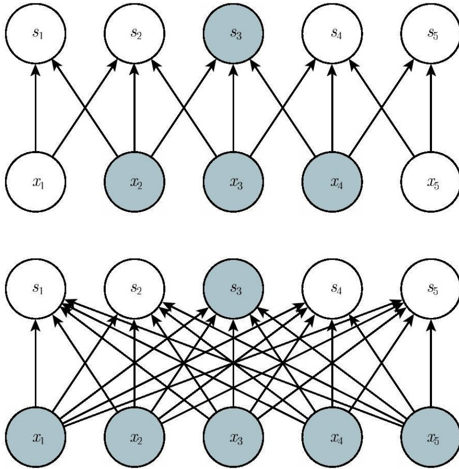
图9.3 稀疏连接，对每幅图从上往下看。我们强调了一个输出单元 s_3 以及 x 中影响该单元的输入单元。这些单元被称为 s_3 的接受域（receptive field）。（上）当 s 是由核宽度为3的卷积产生时，只有3个输入影响 s_3 。（下）当 s 是由矩阵乘法产生时，连接不再是稀疏的，所以所有的输入都会影响 s_3
