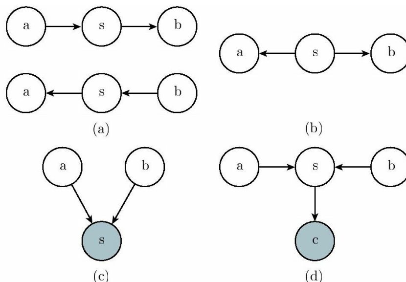
图16.8 两个随机变量 a 和 b 之间存在长度为2的所有种类的活跃路径。(a) 箭头方向从 a 指向 b 的任何路径，反过来也一样。如果 s 可以被观察到，这种路径就是阻塞的。在接力赛的例子中，我们已经看到过这种类型的路径。(b) 变量 a 和 b 通过共因 s 相连。举个例子，假设 s 是一个表示是否存在飓风的变量， a 和 b 表示两个相邻气象监控区域的风速。如果我们在 a 处观察到很高的风速，我们可以期望在 b 处也观察到高速的风。如果观察到 s ，那么这条路径就被阻塞了。如果我们已经知道存在飓风，那么无论 a 处观察到什么，我们都能期望 b 处有较高的风速。在 a 处观察到一个低于预期的风速（对飓风而言）并不会改变我们对 b 处风速的期望（已知有飓风的情况下）。然而，如果 s 不被观测到，那么 a 和 b 是依赖的，即路径是活跃的。(c) 变量 a 和 b 都是 s 的父节点。这称为 V-结构 ( V-structure ) 或者 碰撞情况 ( the collider case )。根据 相消解释作用 ( explaining away effect )，V-结构导致 a 和 b 是相关的。在这种情况下，当 s 被观测到时，路径是活跃的。举个例子，假设 s 是一个表示你的同事不在工作的变量。变量 a 表示她生病了，而变量 b 表示她在休假。如果你观察到了她不在工作，你可以假设她很有可能是生病了或者是在度假，但是这两件事同时发生是不太可能的。如果你发现她在休假，那么这个事实足够解释她的缺席了。你可以推断她很可能没有生病。(d) 即使 s 的任意后代都被观察到，相消解释作用也会起作用。举个例子，假设 c 是一个表示你是否收到你同事的报告的一个变量。如果你注意到你还没有收到这个报告，这会增加你估计的她今天不在工作的概率，这反过来又会增加她今天生病或者度假的概率。阻塞V-结构中路径的唯一方法就是共享子节点的后代一个都观察不到
