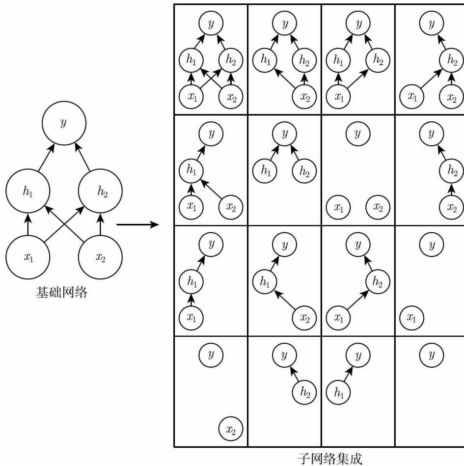
图7.6 Dropout训练由所有子网络组成的集成，其中子网络通过从基本网络中删除非输出单元构建。我们从具有两个可见单元和两个隐藏单元的基本网络开始。这4个单元有16个可能的子集。右图展示了从原始网络中丢弃不同的单元子集而形成的所有16个子网络。在这个小例子中，所得到的大部分网络没有输入单元或没有从输入连接到输出的路径。当层较宽时，丢弃所有从输入到输出的可能路径的概率变小，所以这个问题不太可能在出现层较宽的网络中
