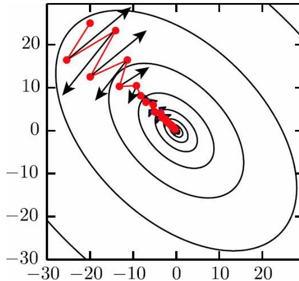
图8.5 动量的主要目的是解决两个问题：Hessian矩阵的病态条件和随机梯度的方差。我们通过此图说明动量如何克服这两个问题的第一个。等高线描绘了一个二次损失函数（具有病态条件的Hessian矩阵）。横跨轮廓的红色路径表示动量学习规则所遵循的路径，它使该函数最小化。在该路径的每个步骤画一个箭头，表示梯度下降将在该点采取的步骤。可以看到，一个病态条件的二次目标函数看起来像一个长而窄的山谷或具有陡峭边的峡谷。动量正确地纵向穿过峡谷，而普通的梯度步骤则会浪费时间在峡谷的窄轴上来回移动。比较图4.6，它也显示了没有动量的梯度下降的行为
