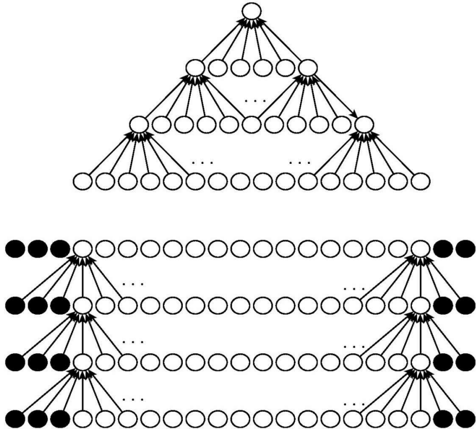
图9.13 零填充对网络大小的影响。考虑一个卷积网络，每层有一个宽度为6的核。在这个例子中，我们不使用任何池化，所以只有卷积操作本身缩小网络的大小。（上）在这个卷积网络中，我们不使用任何隐含的零填充。这使得表示在每层缩小5个像素。从16个像素的输入开始，我们只能有3个卷积层，并且最后一层不能移动核，所以可以说只有两层是真正的卷积层。可以通过使用较小的核来减缓收缩速率，但是较小的核表示能力不足，并且在这种结构中一些收缩是不可避免的。（下）通过向每层添加5个隐含的零，我们防止了表示随深度收缩。这允许我们设计一个任意深的卷积网络
