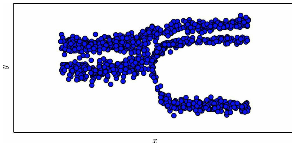
图6.4 从具有混合密度输出层的神经网络中抽取的样本。输入 \mathbf{x} 从均匀分布中采样，输出 y 从 p(\mathbf{model}(y|\mathbf{x})) 中采样。神经网络能够学习从输入到输出分布的参数的非线性映射。这些参数包括控制3个组件中的哪一个将产生输出的概率，以及每个组件各自的参数。每个混合组件都是高斯分布，具有预测的均值和方差。输出分布的 these 方面都能够相对输入 \mathbf{x} 变化，并且以非线性的方式改变
