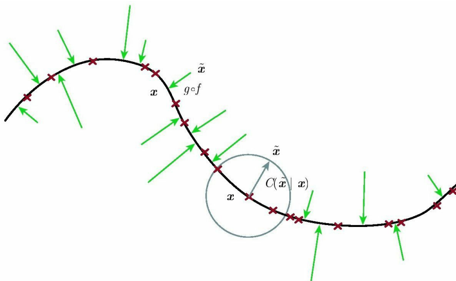
图14.4 去噪自编码器被训练为将损坏的数据点 \tilde{\mathbf{X}} 映射回原始数据点 \mathbf{x} 。我们将训练样本 \mathbf{x} 表为位于低维流形 (粗黑线) 附近的红叉。我们用灰色圆圈表示等概率的损坏过程 C(\tilde{\mathbf{X}} | \mathbf{x}) 。灰色箭头演示了如何将一个训练样本转换为经过此损坏过程的样本。当训练去噪自编码器最小化平方误差 \|g(f(\tilde{\mathbf{x}})) - \mathbf{x}\|^2 的平均值时, 重构 g(f(\tilde{\mathbf{X}})) 估计 \mathbb{E}_{\mathbf{x}, \tilde{\mathbf{x}} \sim p_{\text{data}}(\mathbf{x}) C(\tilde{\mathbf{x}} | \mathbf{x})} [\mathbf{x} | \tilde{\mathbf{x}}] 。对可能产生 \tilde{\mathbf{X}} 的原始点 \mathbf{x} 的质心进行估计, 所以向量 g(f(\tilde{\mathbf{X}})) - \tilde{\mathbf{X}} 近似指向流形上最近的点。因此自编码器可以学习由绿色箭头表示
