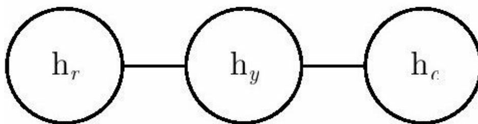
图16.3 表示你室友健康状况的 h_r 、你健康状况的 h_y 和你同事健康状况的 h_c 之间如何相互影响的一个无向图。你和你的室友可能会相互传染感冒，你和你的同事之间也是如此，但是假设你室友和同事之间相互不认识，他们只能通过你来间接传染
