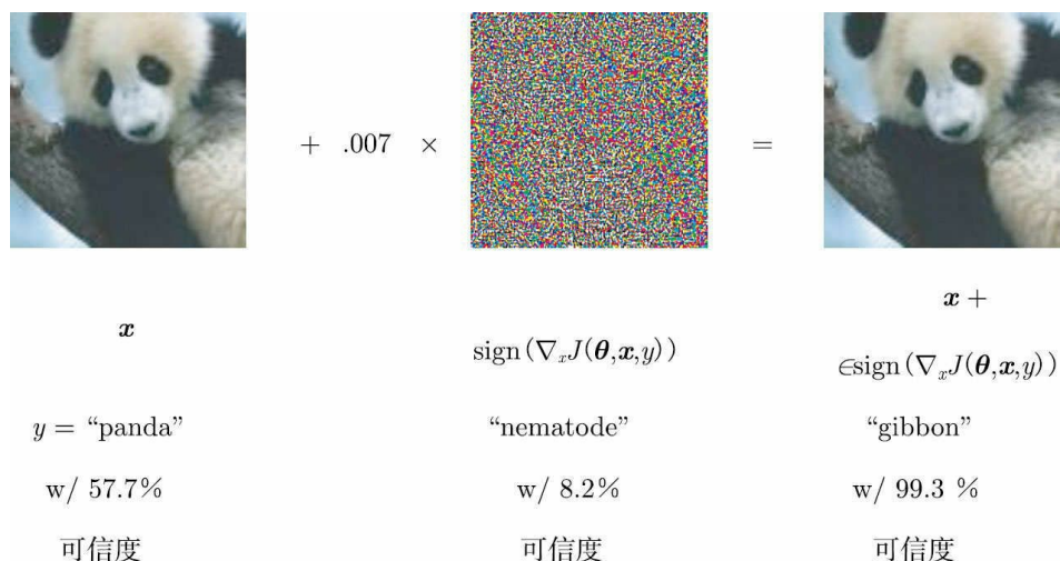
图7.8 在ImageNet上应用GoogLeNet (Szegedy et al. , 2014a) 的对抗样本生成的演示。通过添加一个不可察觉的小向量（其中元素等于代价函数相对于输入的梯度元素的符号），我们可以改变GoogLeNet对此图像的分类结果。经Goodfellow et al. (2014b) 许可转载
