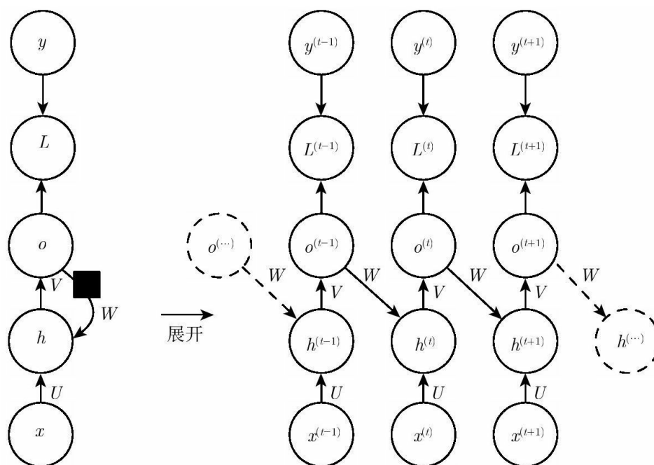
图10.4 此类RNN的唯一循环是从输出到隐藏层的反馈连接。在每个时间步 t ，输入为 x_t ，隐藏层激活为 h^{(t)} ，输出为 o^{(t)} ，目标为 y^{(t)} ，损失为 L^{(t)} 。（左）回路原理图。（右）展开的计算图。这样的RNN没有图10.3表示的RNN那样强大（只能表示更小的函数集合）。图10.3中的RNN可以选择将其想要的关于过去的任何信息放入隐藏表示 h 中并且将 h 传播到未来。该图中的RNN被训练为将特定输出值放入 o 中，并且 o 是允许传播到未来的唯一信息。此处没有从 h 向传播的直接连接。之前的 h 仅通过产生的预测间接地连接到当前。 o 通常缺乏过去的重要信息，除非它非常高维且内容丰富。这使得该图中的RNN不那么强大，但是它更容易训练，因为每个时间步可以与其他时间步分离训练，允许训练期间更多的并行化，如第10.2.1节所述
