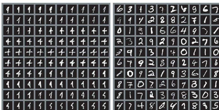
图17.2 深度概率模型中一个混合缓慢问题的例证。每张图都是按照从左到右从上到下的顺序的。（左）Gibbs采样从MNIST数据集训练成的深度玻尔兹曼机中采出的连续样本。这些连续的样本之间非常相似。由于Gibbs采样作用于一个深度图模型，相似度更多地是基于语义而非原始视觉特征。但是对于吉布斯链来说从分布的一个峰值转移到另一个仍然是很困难的，比如说改变数字。（右）从生成式对抗网络中抽出的连续原始样本。因为原始采样生成的样本之间互相独立，所以不存在混合问题
