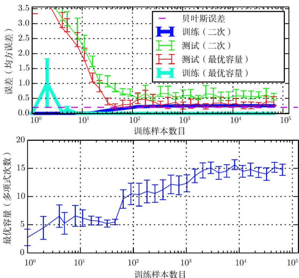
图5.4 训练集大小对训练误差、测试误差以及最优容量的影响。通过给一个5阶多项式添加适当大小的噪声，我们构造了一个合成的回归问题，生成单个测试集，然后生成一些不同尺寸的训练集。为了描述95%置信区间的误差条，对于每一个尺寸，我们生成了40个不同的训练集。（上）两个不同的模型上训练集和测试集的MSE，一个二次模型，另一个模型的阶数通过最小化测试误差来选择。两个模型都是用闭式解来拟合。对于二次模型来说，当训练集增加时，训练误差也随之增大。这是由于越大的数据集越难以拟合。同时，测试误差随之减小，因为关于训练数据的不正确的假设越来越少。二次模型的容量并不足以解决这个问题，所以它的测试误差趋近于一个较高的值。最优容量点处的测试误差趋近于贝叶斯误差。训练误差可以低于贝叶斯误差，因为训练算法有能力记住训练集中特定的样本。当训练集趋向于无穷大时，任何固定容量的模型（在这里指的是二次模型）的训练误差都至少增至贝叶斯误差。（下）当训练集大小增大时，最优容量（在这里是用最优多项式回归器的阶数衡量的）也会随之增大。最优容量在达到足够捕捉模型复杂度之后就不再增长了
