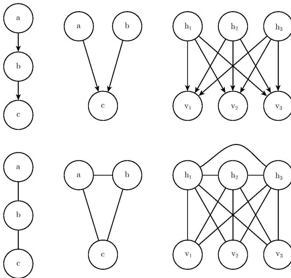
图16.11 通过构造道德图将有向模型（上一行）转化为无向模型（下一行）的例子。（左）只需要把有向边替换成无向边就可以把这个简单的链转化为一个道德图。得到的无向模型包含了完全相同的独立关系和条件独立关系。（中）是在不丢失独立性的情况下无法转化为无向模型的最简单的有向模型。这个图包含了单个完整的不道德结构。因为a和b都是c的父节点，当c被观察到时，它们之间通过活跃路径相连。为了捕捉这个依赖，无向模型必须包含一个含有所有三个变量的团。这个团无法编码 a \perp b 这个信息。（右）一般来说，道德化的过程会给图添加许多边，因此丢失了一些隐含的独立性。举个例子，这个稀疏编码图需要在每一对隐藏单元之间添加道德化的边，因此也引入了二次数量级的新的直接依赖
