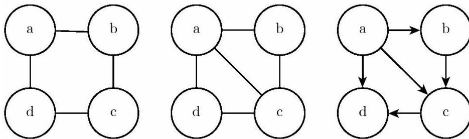
图16.12 将一个无向模型转化为一个有向模型。(左) 这个无向模型无法转化为有向模型, 因为它有一个长度为4且不带有弦的环。具体说来, 这个无向模型包含了两种不同的独立性, 并且不存在一个有向模型可以同时描述这两种性质: a \perp c \mid \{b, d\} 和 b \perp d \mid \{a, c\} 。(中) 为了将无向图转化为有向图, 我们必须通过保证所有长度大于3的环都有弦来三角形化图。为了实现这个目标, 我们可以加一条连接a和c或者连接b和d的边。在这个例子中, 我们选择添加一条连接a和c的边。(右) 为了完成转化的过程, 我们必须给每条边分配一个方向。执行这个任务时, 我们必须保证不产生任何有向环。避免出现有向环的一种方法是赋予节点一定的顺序, 然后将每个边从排序较早的节点指向排序稍后的节点。在这个例子中, 我们根据变量名的字母进行排序
