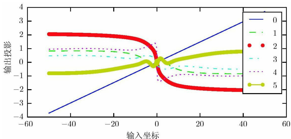
图10.15 重复组合函数。当组合许多非线性函数（如这里所示的线性tanh层）时，结果是高度非线性的，通常大多数值与微小的导数相关联，也有一些具有大导数的值，以及在增加和减小之间的多次交替。此处，我们绘制从100维隐藏状态降到单个维度的线性投影，绘制于y轴上。x轴是100维空间中沿着随机方向的初始状态的坐标。因此，我们可以将该图视为高维函数的线性截面。曲线显示每个时间步之后的函数，或者等价地，转换函数被组合一定次数之后
