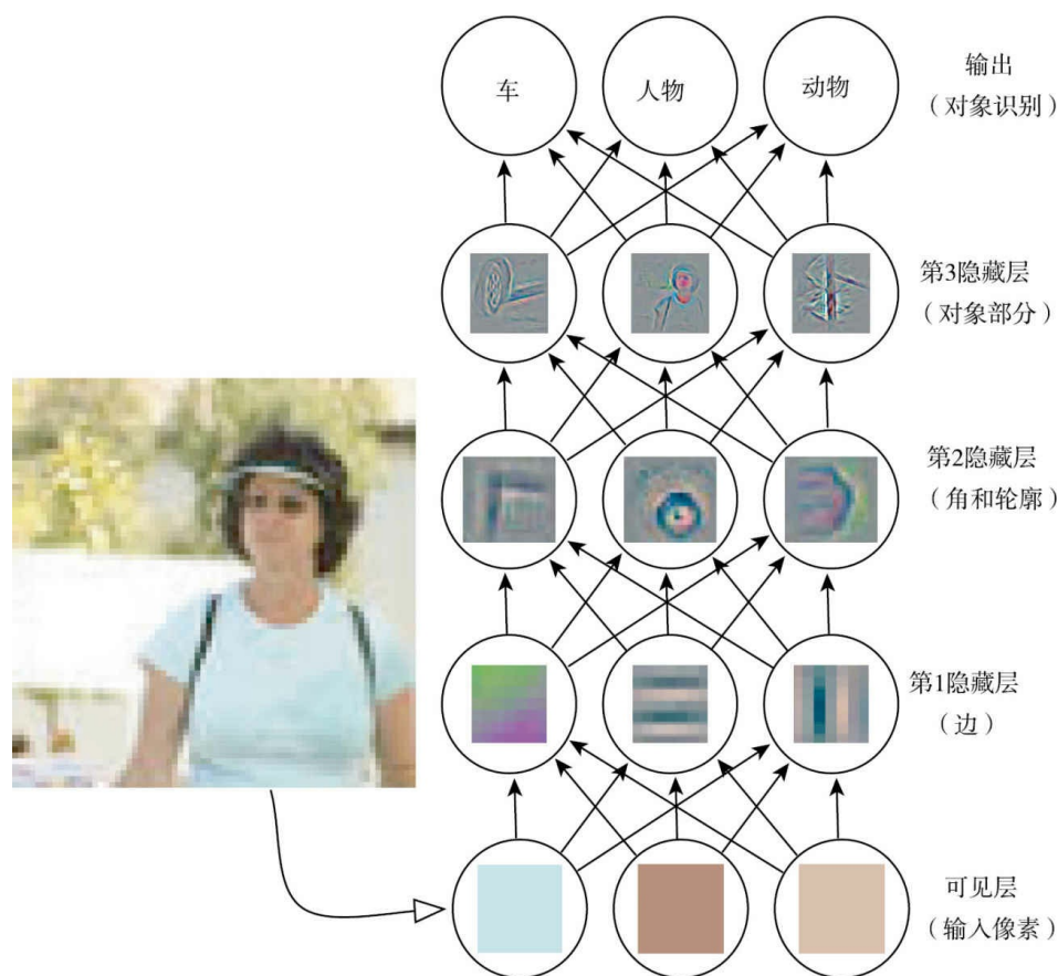
图1.2 深度学习模型的示意图。计算机难以理解原始感观输入数据的含义，如表示为像素值集合的图像。将一组像素映射到对象标识的函数非常复杂。如果直接处理，学习或评估此映射似乎是不可能的。深度学习将所需的复杂映射分解为一系列嵌套的简单映射（每个由模型的不同层描述）来解决这一难题。输入展示在可见层（visible layer），这样命名的原因是因为它包含我们能观察到的变量。然后是一系列从图像中提取越来越多抽象特征的隐藏层（hidden layer）。因为它们的值不在数据中给出，所以将这些层称为“隐藏层”；模型必须确定哪些概念有利于解释观察数据中的关系。这里的图像是每个隐藏单元表示的特征的可视化。给定像素，第1层可以轻易地通过比较相邻像素的亮度来识别边缘。有了第1隐藏层描述的边缘，第2隐藏层可以容易地搜索可识别为角和扩展轮廓的边集合。给定第2隐藏层中关于角和轮廓的图像描述，第3隐藏层可以找到轮廓和角的特定集合来检测特定对象的整个部分。最后，根据图像描述中包含的对象部分，可以识别图像中存在的对象（经Zeiler and Fergus（2014）许可引用此图）
