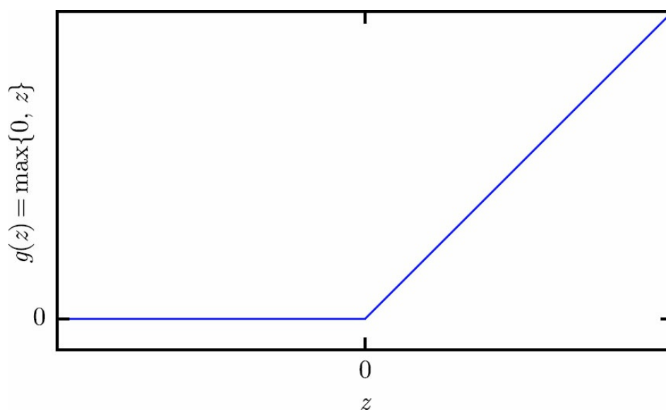
图6.3 整流线性激活函数。该激活函数是被推荐用于大多数前馈神经网络的默认激活函数。将此函数用于线性变换的输出将产生非线性变换。然而，函数仍然非常接近线性，在这种意义上它是具有两个线性部分的分段线性函数。由于整流线性单元几乎是线性的，因此它们保留了许多使得线性模型易于使用基于梯度的方法进行优化的属性。它们还保留了许多使得线性模型能够泛化良好的属性。计算机科学的一个公共原则是，我们可以从最小的组件构建复杂的系统。就像图灵机的内存只需要能够存储0或1的状态，我们可以从整流线性函数构建一个万能函数近似器
