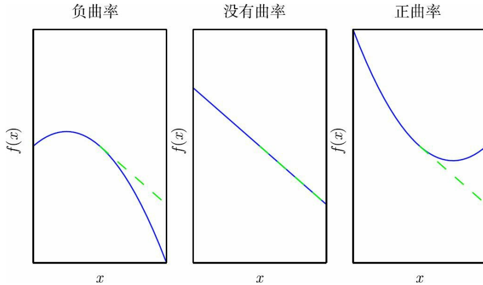
图4.4 二阶导数确定函数的曲率。这里我们展示具有各种曲率的二次函数。虚线表示我们仅根据梯度信息进行梯度下降后预期的代价函数值。对于负曲率，代价函数实际上比梯度预测下降得更快。没有曲率时，梯度正确预测下降值。对于正曲率，代价函数比预期下降得更慢，并且最终会开始增加，因此太大的步骤实际上可能会无意地增加函数值
