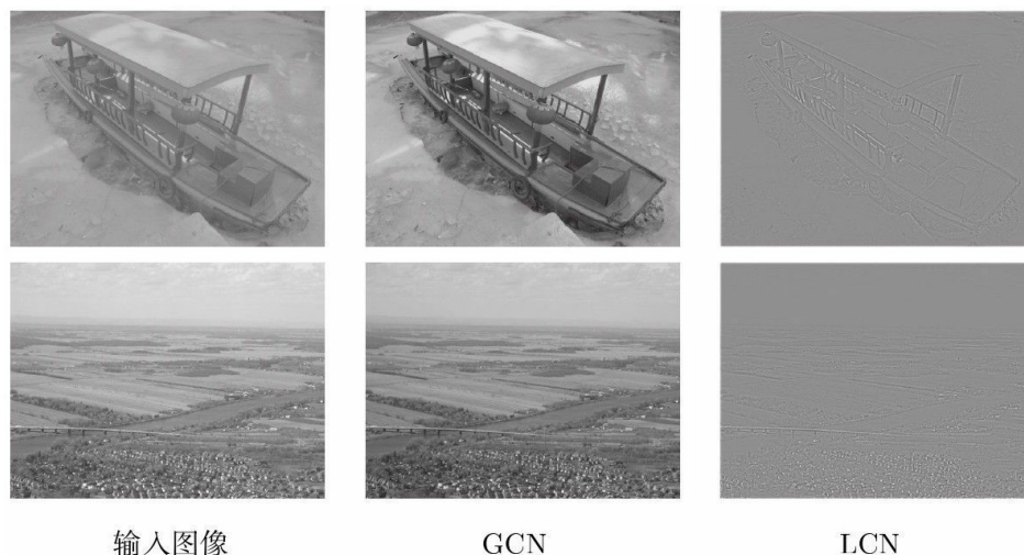
图12.2 全局对比度归一化和局部对比度归一化的比较。直观上说，全局对比度归一化的效果很巧妙。它使得所有图片的尺度都差不多，这减轻了学习算法处理多个尺度的负担。局部对比度归一化更多地改变了图像，丢弃了所有相同强度的区域。这使模型能够只关注于边缘。较好的纹理区域，如第二行的屋子，可能会由于归一化核的过高带宽而丢失一些细节
