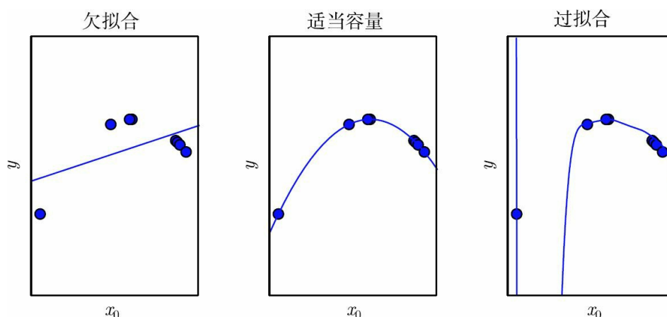
图5.2 我们用3个模型拟合了这个训练集的样本。训练数据是通过随机抽取 x 然后用二次函数确定性地生成 y 来合成的。（左）用一个线性函数拟合数据会导致欠拟合——它无法捕捉数据中的曲率信息。（中）用二次函数拟合数据在未观察到的点上泛化得很好，这并不会导致明显的欠拟合或者过拟合。（右）一个9阶的多项式拟合数据会导致过拟合。在这里我们使用Moore-Penrose伪逆来解这个欠定的正规方程。得出的解能够精确地穿过所有的训练点，但可惜我们无法提取有效的结构信息。在两个数据点之间它有一个真实的函数所不包含的深谷。在数据的左侧，它也会急剧增长，而在这一区域真实的函数却是下降的
