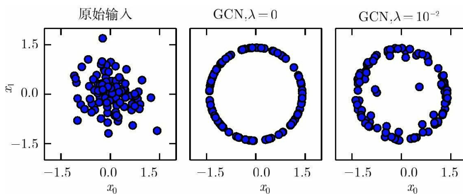
图12.1 GCN将样本投影到一个球上。（左）原始的输入数据可能拥有任意的范数。（中） \lambda=0 时，GCN可以完美地将所有的非零样本投影到球上。这里我们令 s=1 ， \epsilon=10^{-8} 。由于我们使用的GCN是基于归一化标准差而不是 L^2 范数，所得到的球并不是单位球。（右） \lambda>0 的正则化GCN将样本投影到球上，但是并没有完全地丢弃其范数中变化。 s 和 \epsilon 的取值与之前一样
