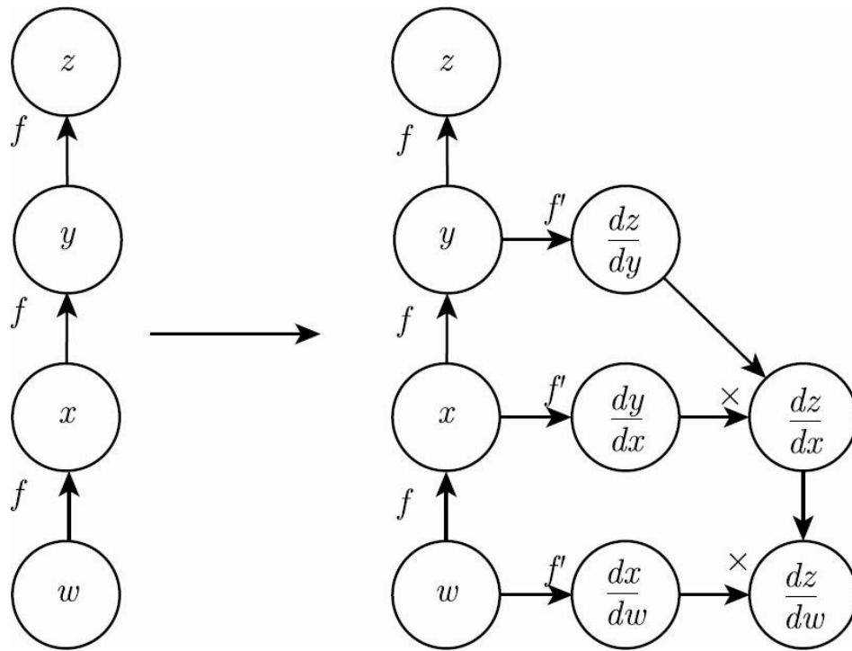
图6.10 使用符号到符号的方法计算导数的示例。在这种方法中，反向传播算法不需要访问任何实际的特定数值。相反，它将节点添加到计算图中来描述如何计算这些导数。通用图形求值引擎可以在随后计算任何特定数值的导数。（左）在这个例子中，我们从表示 z=f(f(f(w))) 的计算图开始。（右）我们运行反向传播算法，指导它构造表达式 \frac{dz}{dw} 对应的图。在这个例子中，我们不解释反向传播算法如何工作。我们的目的只是说明想要的结果是什么：符号描述的导数的计算图
