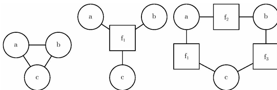
图16.13 因子图如何解决无向网络中模糊性的一个例子。（左）一个包含3个变量（a、b和c）的团组成的无向网络。（中）对应这个无向模型的因子图。这个因子图有一个包含3个变量的因子。（右）对应这个无向模型的另一种有效的因子图。这个因子图包含了3个因子，每个因子只对应两个变量。即使它们表示的是同一个无向模型，这个因子图上进行的表示、推断和学习相比于中图描述的因子图都要渐近地廉价
