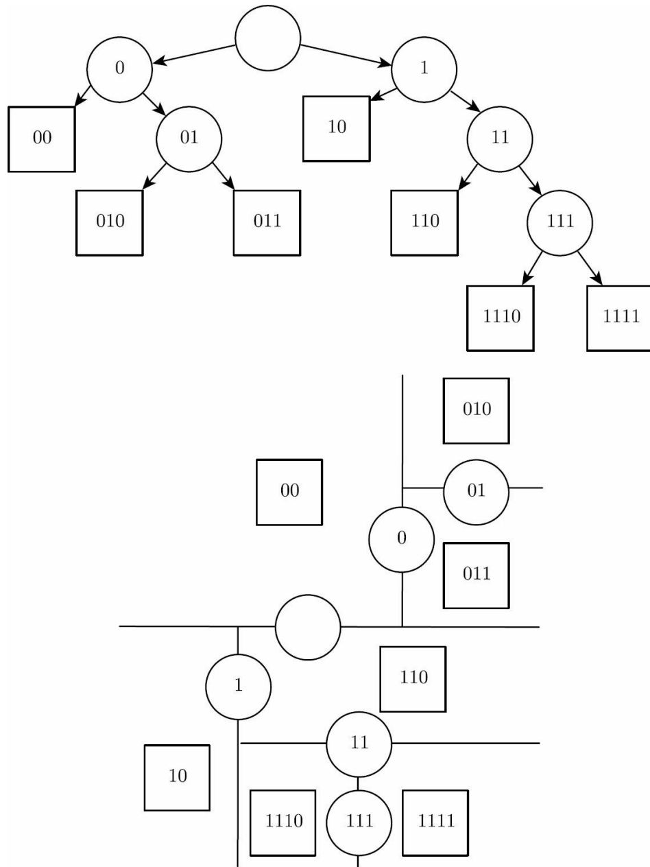
图5.7 描述一个决策树如何工作的示意图。（上）树中每个节点都选择将输入样本送到左子节点（0）或者右子节点（1）。内部的节点用圆圈表示，叶节点用方块表示。每一个节点可以用一个二值的字符串识别并对应树中的位置，这个字符串是通过给起父亲节点的字符串添加一个位元来实现的（0表示选择左或者上，1表示选择右或者下）。（下）这个树将空间分为区域。这个二维平面说明决策树可以分割 \mathbb{R}^2 。这个平面中画出了树的节点，每个内部点穿过分割线并用来给样本分类，叶节点画在样本所属区域的中心。结果是一个分块常数函数，每一个叶节点一个区域。每个叶需要至少一个训练样本来定义，所以决策树不可能用来学习一个局部极大值比训练样本数量还多的函数
