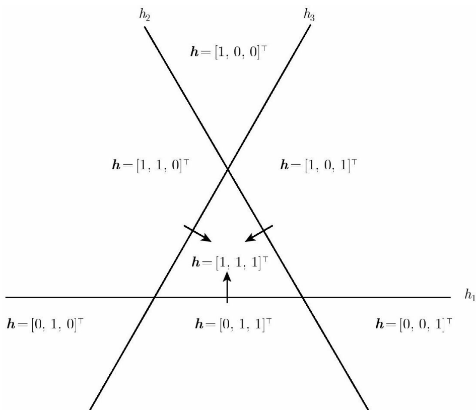
图15.7 基于分布式表示的学习算法如何将输入空间分割成多个区域的图示。这个例子具有二元变量 h_1 、 h_2 、 h_3 。每个特征通过为学成的线性变换设定输出阈值而定义。每个特征将 \mathbb{R}^2 分成两个半平面。令 h_i^+ 表示输入点 h_i=1 的集合； h_i^- 表示输入点 h_i=0 的集合。在这个图中，每条线代表着一个 h_i 的决策边界，对应的箭头指向边界的 h_i^+ 区域。整个表示在这些半平面的每个相交区域都指定一个唯一值。例如，表示值为 [1, 1, 1]^T 对应着区域 h_1^+ \cap h_2^+ \cap h_3^+ 。可以将以上表示和图15.8中的非分布式表示进行比较。在输入维度是 d 的一般情况下，分布式表示通过半空间（而不是半平面）的交叉分割 \mathbb{R}^d 。具有 n 个特征的分布式表示给 O(2^n) 个不同区域分配唯一的编码，而具有 n 个样本的最近邻算法只能给 n 个不同区域分配
