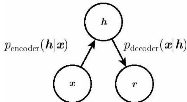
图14.2 随机自编码器的结构，其中编码器和解码器包括一些噪声注入，而不是简单的函数。这意味着可以将它们的输出视为来自分布的采样（对于编码器是 p_{\text{encoder}}(\mathbf{h} | \mathbf{x}) ，对于解码器是 p_{\text{decoder}}(\mathbf{x} | \mathbf{h}) ）
