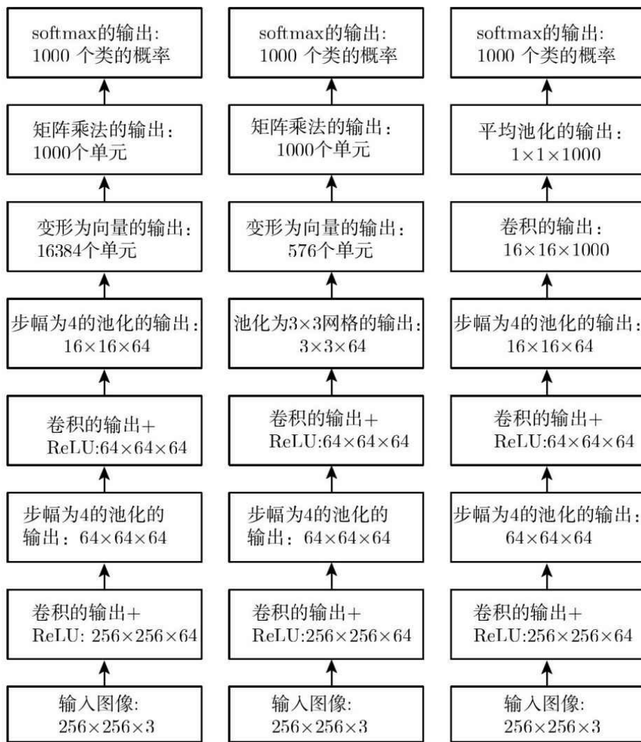
图9.11 卷积网络用于分类的结构示例。本图中使用的具体步幅和深度并不建议实际使用，因为它们被设计得非常浅以适合页面。实际的卷积网络还常常涉及大量的分支，不同于这里为简单起见所使用的链式结构。（左）处理固定大小的图像的卷积网络。在卷积层和池化层几层交替之后，卷积特征映射的张量被重新变形以展平空间维度。网络的其余部分是一个普通的前馈网络分类器，如第6章所述。（中）处理大小可变的图像的卷积网络，但仍保持全连接的部分。该网络使用具有可变大小但是数量固定的池的池化操作，以便向网络的全连接部分提供固定576个单位大小的向量。（右）没有任何全连接权重层的卷积网络。相对的，最后的卷积层为每个类输出一个特征映射。该模型可能会用来学习每个类出现在每个空间位置的可能性的映射。将特征映射进行平均得到的单个值，提供了顶部softmax分类器的变量
