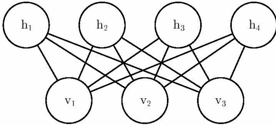
图16.14 一个画成马尔可夫网络形式的RBM
