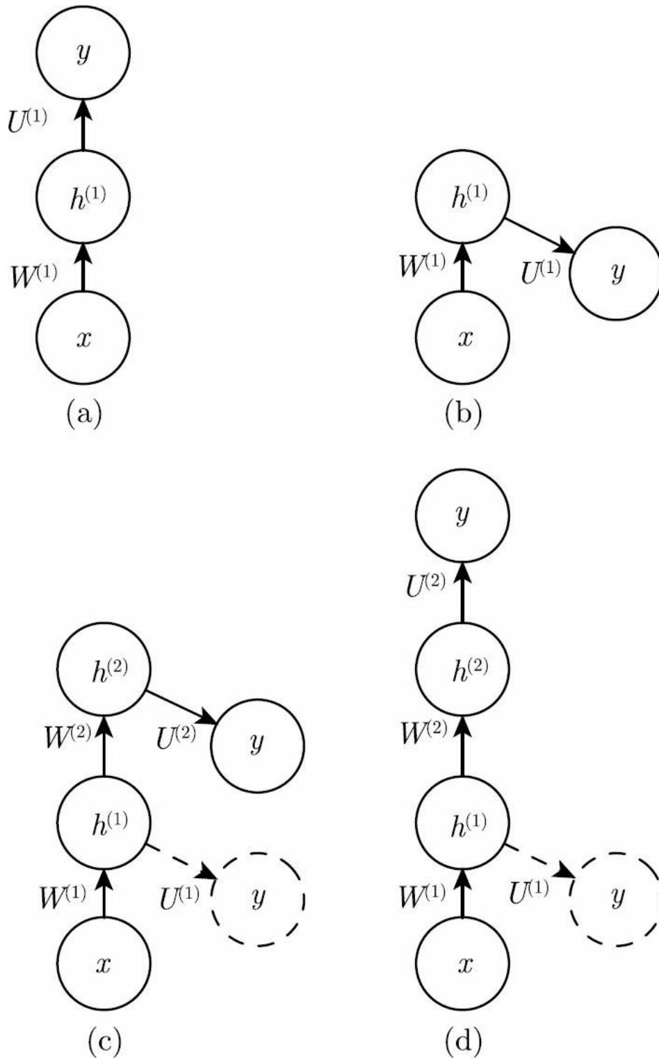
图8.7 一种形式的贪心监督预训练的示意图 (Bengio et al. , 2007a)。(a) 我们从训练一个足够浅的架构开始。(b) 同一个架构的另一描绘。(c) 我们只保留原始网络的输入到隐藏层, 并丢弃隐藏到输出层。我们将第一层隐藏层的输出作为输入发送到另一监督单隐层MLP (使用与第一个网络相同的目标训练), 从而可以添加第二层隐藏层。这可以根据需要重复多层。
