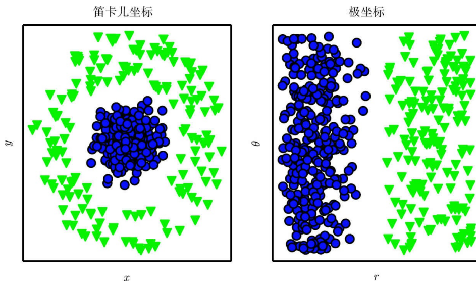
图1.1 不同表示的例子：假设我们想在散点图中画一条线来分隔两类数据。在左图中，我们使用笛卡儿坐标表示数据，这个任务是不可能的。在右图中，我们用极坐标表示数据，可以用垂直线简单地解决这个任务（与David Warde-Farley合作绘制此图）
