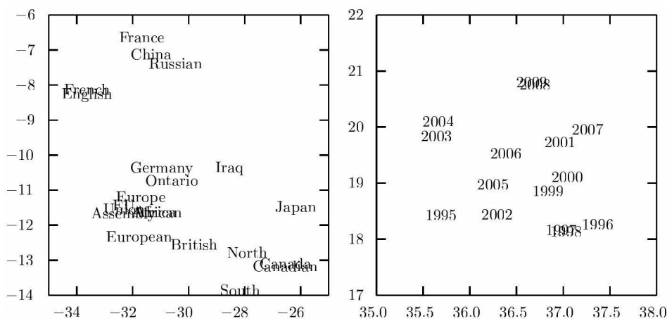
图12.3 从神经机器翻译模型获得的词嵌入的二维可视化（Bahdanau et al. ，2015）。此图在语义相关词的特定区域放大，它们具有彼此接近的嵌入向量。国家在左图，数字在右图。注意，这些嵌入是为了可视化才表示为二维。在实际应用中，嵌入通常具有更高的维度并且可以同时捕获词之间多种相似性
