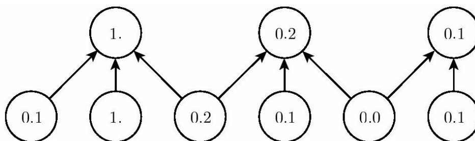
图9.10 带有降采样的池化。这里我们使用最大池化，池的宽度为三并且池之间的步幅为二。这使得表示的大小减少了一半，减轻了下一层的计算和统计负担。注意到最右边的池化区域尺寸较小，但如果我们不想忽略一些探测单元，就必须包含这个区域
