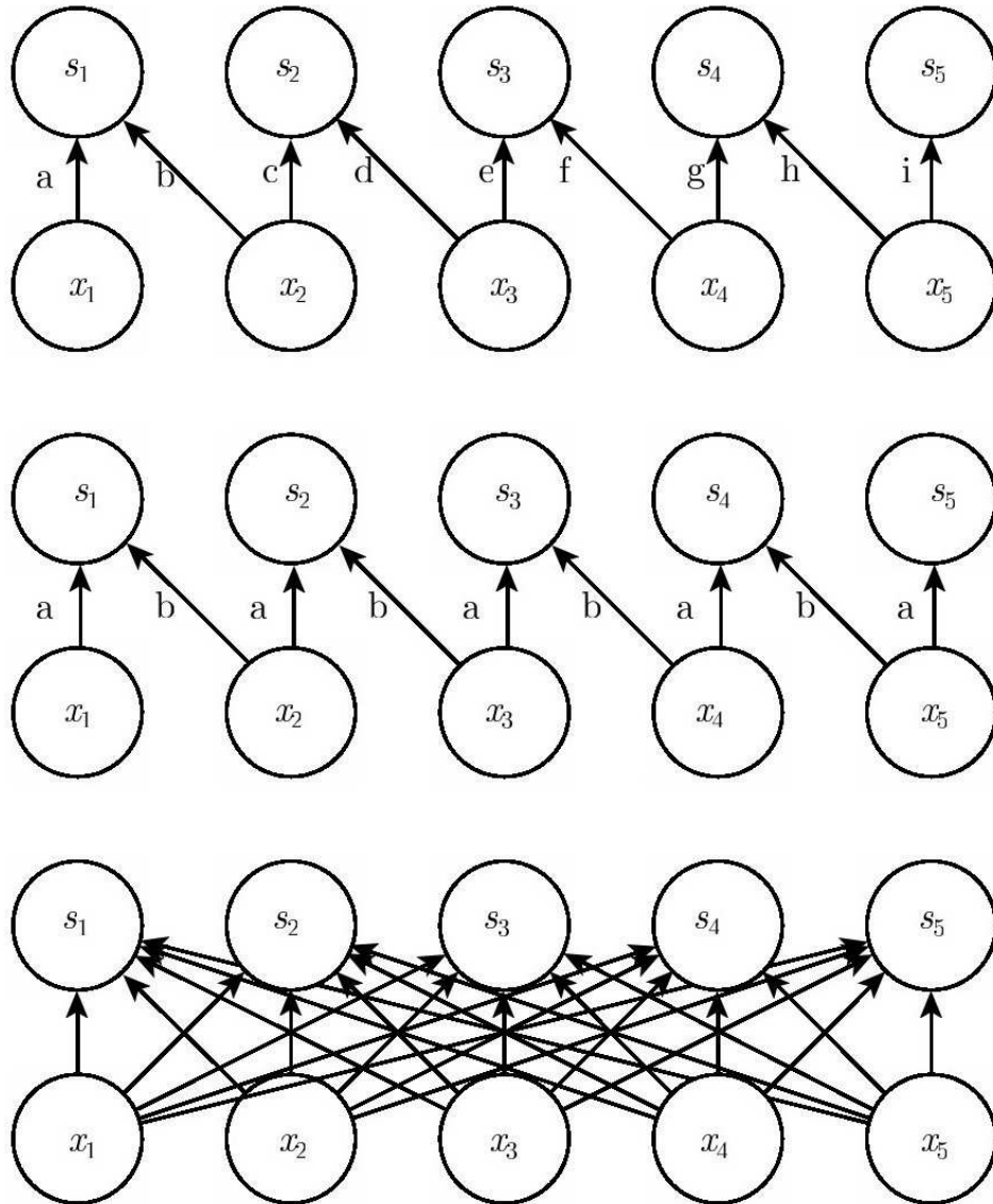
图9.14 局部连接，卷积和全连接的比较。（上）每一小片（接受域）有两个像素的局部连接层。每条边用唯一的字母标记，来显示每条边都有自身的权重参数。（中）核宽度为两个像素的卷积层。该模型与局部连接层具有完全相同的连接。区别不在于哪些单元相互交互，而在于如何共享参数。局部连接层没有参数共享。正如用于标记每条边的字母重复出现所指示的，卷积层在整个输入上重复使用相同的两个权重。（下）全连接层类似于局部连接层，它的每条边都有其自身的参数（在该图中用字母明确标记就太多了）。然而，它不具有局部连接层的连接受限的特征
