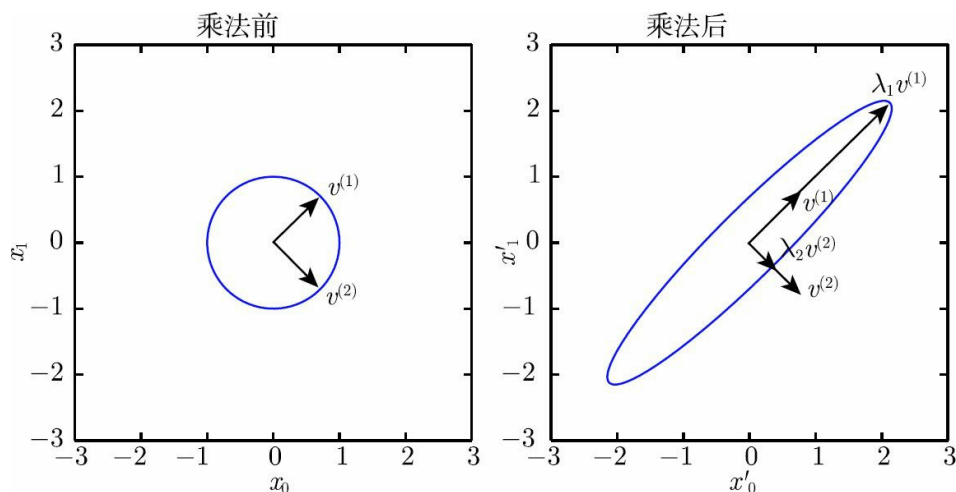
图2.3 特征向量和特征值的作用效果。特征向量和特征值的作用效果的一个实例。在这里，矩阵 \mathbf{A} 有两个标准正交的特征向量，对应特征值为 \lambda_1 的 \mathbf{v}^{(1)} 以及对应特征值为 \lambda_2 的 \mathbf{v}^{(2)} 。
