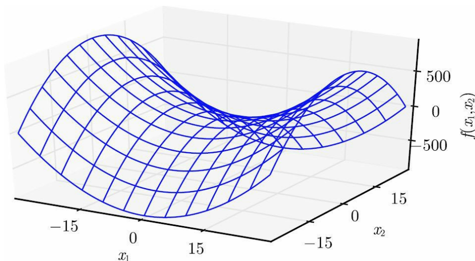
图4.5 既有正曲率又有负曲率的鞍点。示例中的函数是 f(x) = x_1^2 - x_2^2 。函数沿 x_1 轴向上弯曲。 x_1 轴是Hessian的一个特征向量，并且具有正特征值。函数沿 x_2 轴向下弯曲。该方向对应于Hessian负特征值的特征向量。名称“鞍点”源自该处函数的鞍状形状。这是具有鞍点函数的典型示例。维度多于一个时，鞍点不一定要具有0特征值：仅需要同时具有正特征值和负特征值。我们可以想象这样一个鞍点（具有正负特征值）在一个横截面内是局部极大点，而在另一
