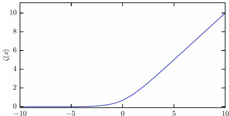
图3.4 softplus函数
