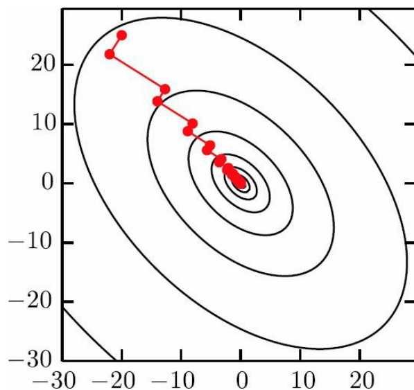
图8.6 将最速下降法应用于二次代价表面。在每个步骤中，最速下降法沿着由初始点处的梯度定义的线跳到最低代价的点。这解决了图4.6中使用固定学习率所遇到的一些问题，但即使使用最佳步长，算法仍然朝最优方向曲折前进。根据定义，在沿着给定方向的目标最小值处，最终点处的梯度与该方向正交
