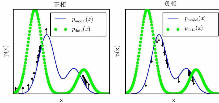
图18.1 算法18.1角度的“正相”和“负相”。（左）在正相中，我们从数据分布中采样，然后推高它们未归一化的概率。这意味着概率越高的数据点，未归一化的概率被推高得越多。（右）在负相中，我们从模型分布中采样，然后压低它们未归一化的概率。这与正相的倾向相反，给未归一化的概率处处添加了一个大常数。当数据分布和模型分布相等时，正相推高数据点和负相压低数据点的机会相等。此时，不再有任何的梯度（期望上说），训练也必须停止
