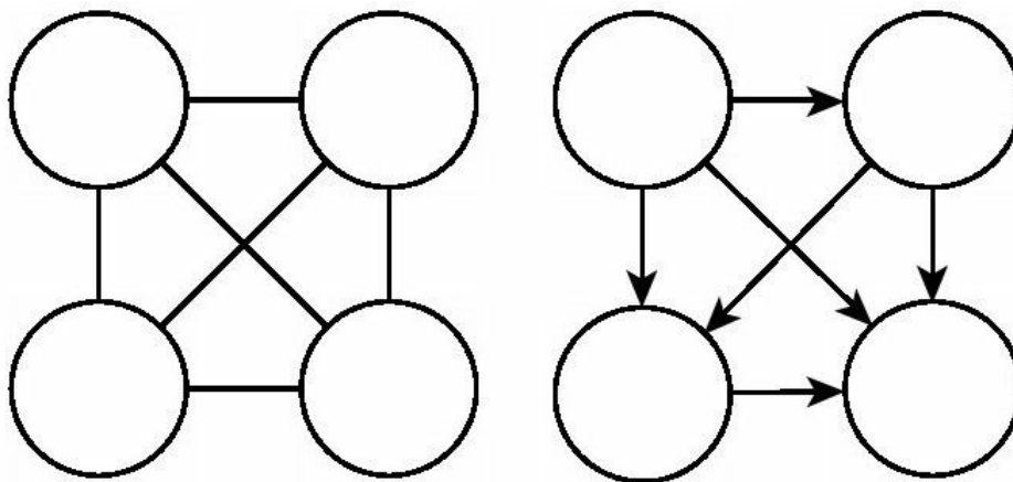
图16.10 完全图的例子，完全图能够描述任何的概率分布。这里我们展示了一个带有4个随机变量的例子。（左）完全无向图。在无向图中，完全图是唯一的。（右）一个完全有向图。在有向图中，并不存在唯一的完全图。我们选择一种变量的排序，然后对每一个变量，从它本身开始，向每一个指向顺序在其后面的变量画一条弧。因此存在着关于变量数阶乘数量级的不同
