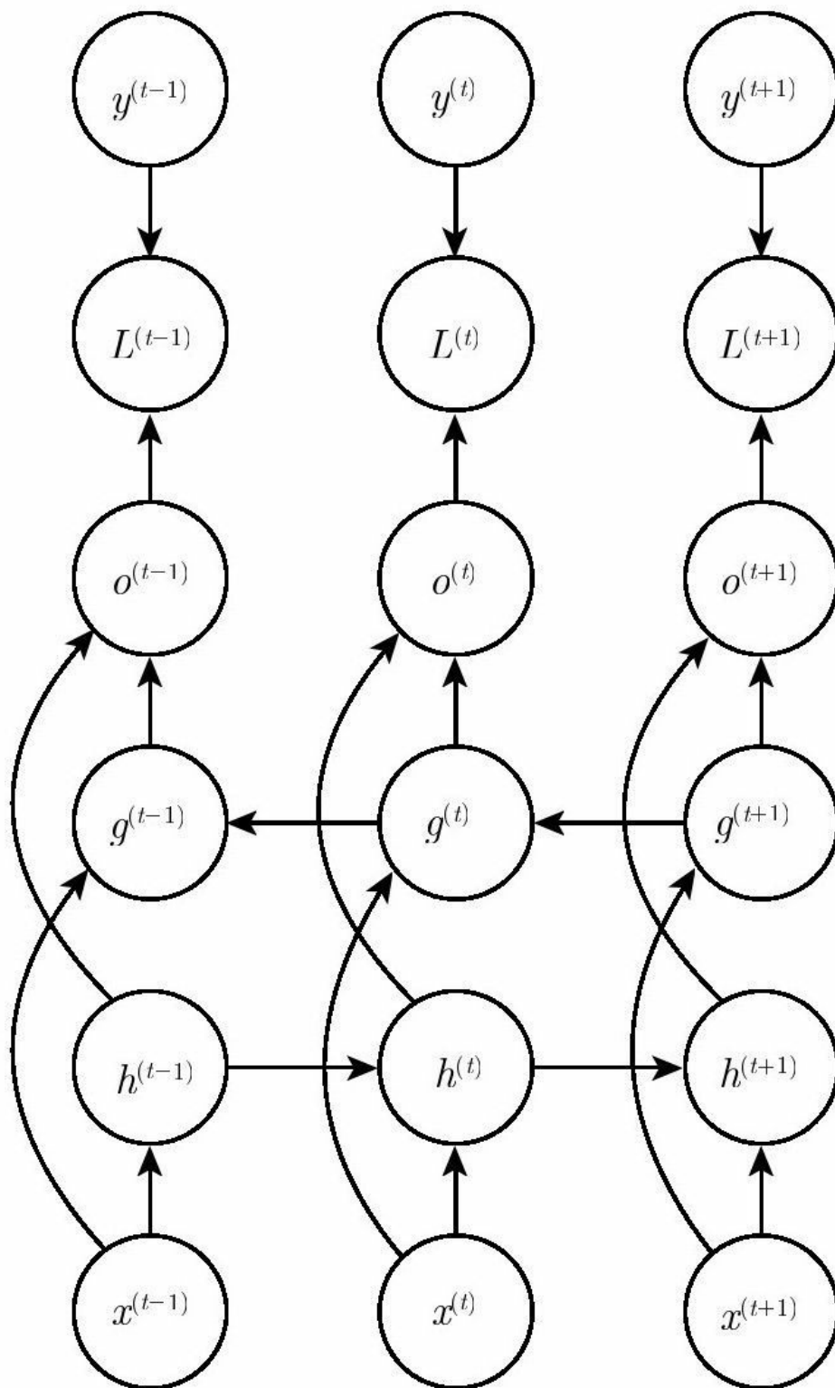
图10.11 典型的双向循环神经网络中的计算，意图学习将输入序列 \mathbf{x} 映射到目标序列 \mathbf{y} （在每个步骤 t 具有损失 L^{(t)} ）。循环性 \mathbf{h} 在时间上向前传播信息（向右），而循环性 \mathbf{g} 在时间上向后
