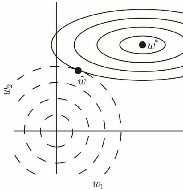
图7.1 L^2 （或权重衰减）正则化对最佳 w 值的影响。实线椭圆表示没有正则化目标的等值线。虚线圆圈表示 L^2 正则化项的等值线。在 \tilde{w} 点，这两个竞争目标达到平衡。目标函数 J 的 Hessian 的第一维特征值很小。当从 w^* 水平移动时，目标函数不会增加得太多。因为目标函数对这个方向没有强烈的偏好，所以正则化项对该轴具有强烈的影响。正则化项将 w_1 拉向零。而目标函数对沿着第二维远离 w^* 的移动非常敏感。对应的特征值较大，表示高曲率。因此，权重衰减对 w_2 的位置影响相对较小。
