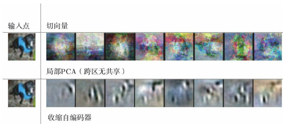
图14.10 通过局部PCA和收缩自编码器估计的流形切向量的图示。流形的位置由来自CIFAR-10数据集中狗的输入图像定义。切向量通过输入到代码映射的Jacobian矩阵 \frac{\partial \mathbf{h}}{\partial \mathbf{x}} 的前导奇异向量估计。虽然局部PCA和CAE都可以捕获局部切方向，但CAE能够从有限训练数据形成更准确的估计，因为它利用了不同位置的参数共享（共享激活的隐藏单元子集）。CAE切方向通常对应于物体的移动或改变部分（例如头或腿）。经Rifai et al. (2011c) 许可转载此图
