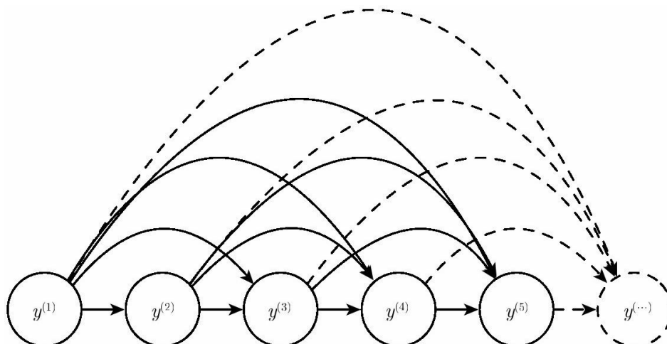
图10.7 序列 y^{(1)}, y^{(2)}, \dots, y^{(t)}, \dots 的全连接图模型。给定先前的值，每个过去的观察值 y^{(i)} 可以影响一些 y^{(t)} ( t > i )的条件分布。当序列中每个元素的输入和参数的数目越来越多，根据此图直接参数化图模型（如式（10.6）中）可能是非常低效的。RNN可以通过高效的参数化获得相同的全连接，如图10.8所示
