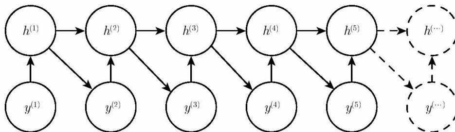
图10.8 在RNN图模型中引入状态变量，尽管它是输入的确定性函数，但它有助于我们根据式（10.5）获得非常高效的参数化。序列中的每个阶段（对于 \mathbf{h}^{(t)} 和 \mathbf{y}^{(t)} ）使用相同的结构（每个节点具有相同数量的输入），并且可以与其他阶段共享相同的参数
