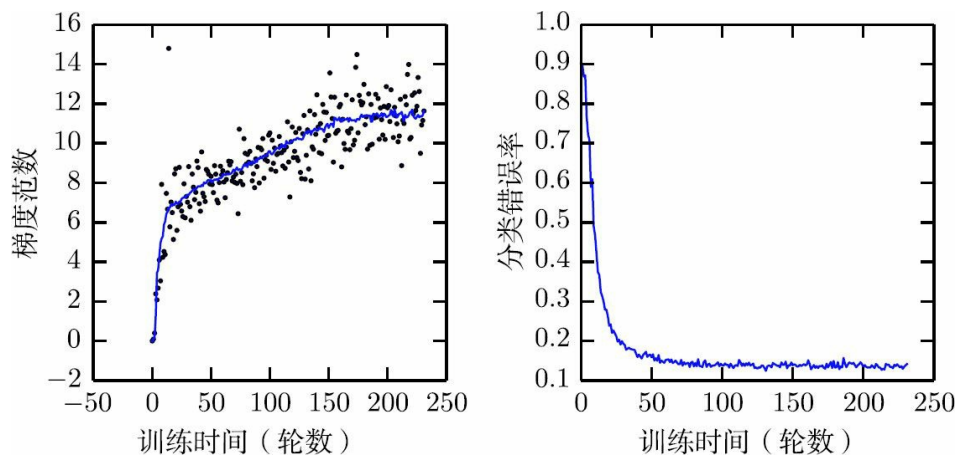
图8.1 梯度下降通常不会到达任何类型的临界点。此示例中，在用于对象检测的卷积网络的整个训练期间，梯度范数持续增加。（左）各个梯度计算的范数如何随时间分布的散点图。为了方便作图，每轮仅绘制一个梯度范数。我们将所有梯度范数的移动平均绘制为实曲线。梯度范数明显随时间增加，而不是如我们所期望的那样随训练过程收敛到临界点而减小。（右）尽管梯度递增，训练过程却相当成功。验证集上的分类误差可以降低到较低水平
