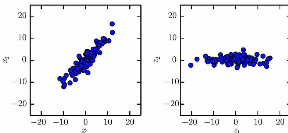
图5.8 PCA学习一种线性投影，使最大方差的方向和新空间的轴对齐。（左）原始数据包含了 \mathbf{x} 的样本。在这个空间中，方差的方向与轴的方向并不是对齐的。（右）变换过的数据 \mathbf{z} = \mathbf{x}^T \mathbf{W} 在轴 z_1 的方向上有最大的变化。第二大变化方差的方向沿着轴 z_2
