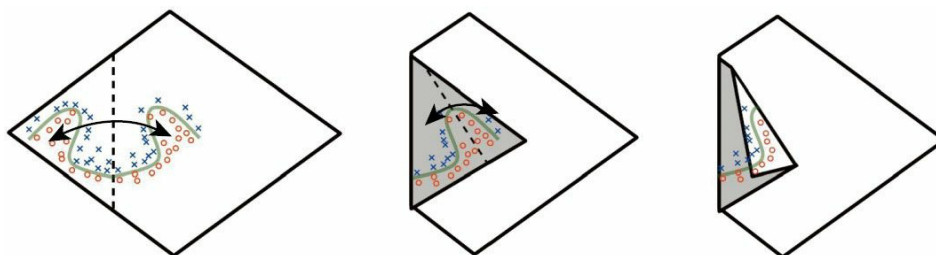
图6.5 关于更深的整流网络具有指数优势的一个直观的几何解释，来自Montufar et al. (2014)。(左)绝对值整流单元对其输入中的每对镜像点有相同的输出。镜像的对称轴由单元的权重和偏置定义的超平面给出。在该单元顶部计算的函数（绿色决策面）将是横跨该对称轴的更简单模式的一个镜像。(中)该函数可以通过折叠对称轴周围的空间来得到。(右)另一个重复模式可以在第一个的顶部折叠（由另一个下游单元）以获得另外的对称性（现在重复4次，使用了两个隐藏层）。经Montufar et al. (2014) 许可引用此图
