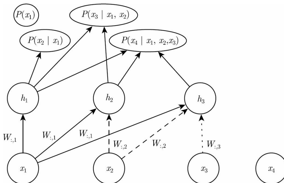
图20.10 神经自回归密度估计器（NADE）的示意图。隐藏单元被组织在组 h^{(i)} 中，使得只有输入 x_1, \dots, x_i 参与计算 h^{(i)} 和预测 P(x_j | x_{j-1}, \dots, x_1) （对于 j > i ）。NADE 用特定的权重共享模式区别于早期的神经自回归网络： W'_{j,k,i} = W_{k,i} 被共享于所有从 x_i 到任
