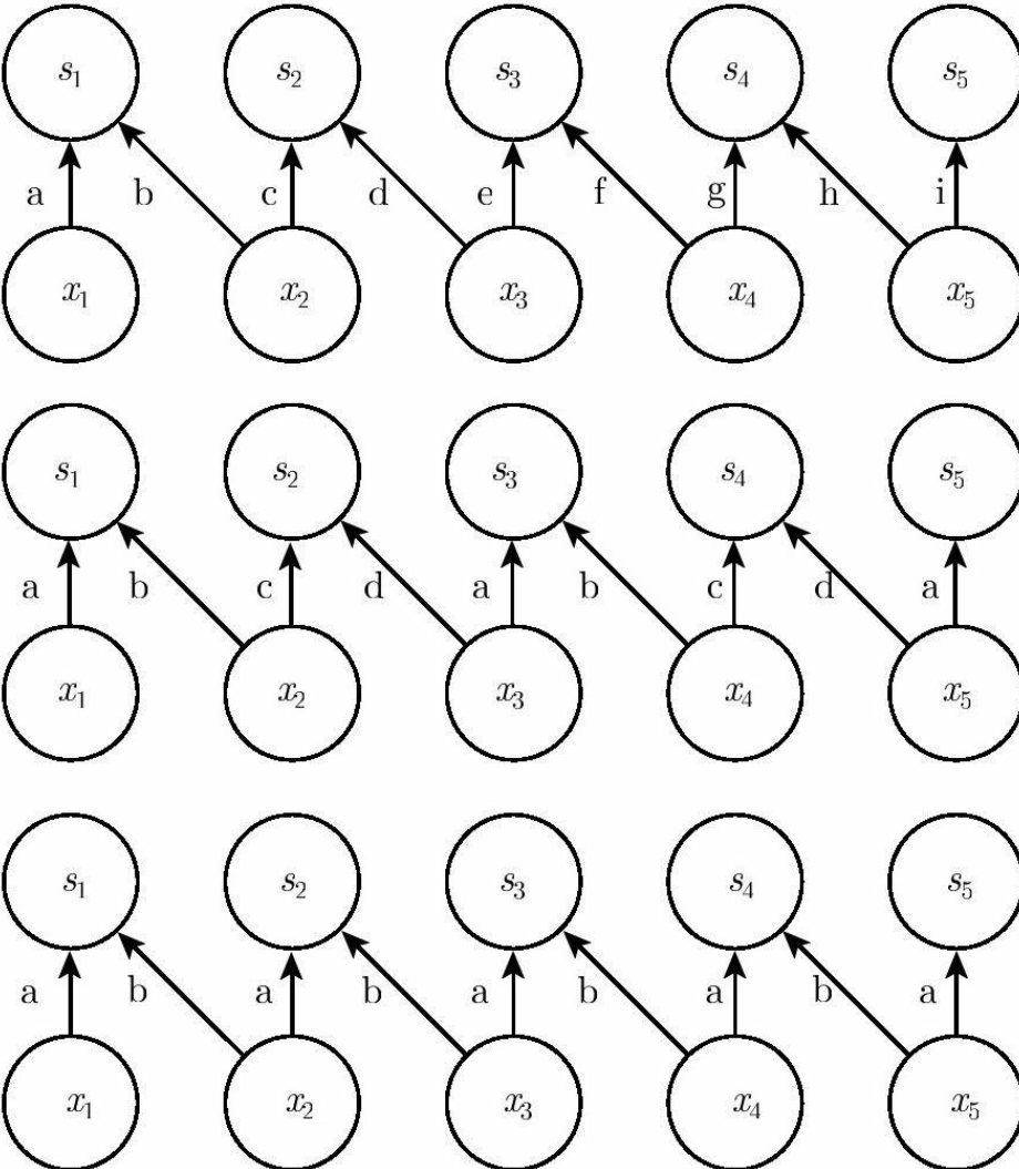
图9.16 局部连接层、平铺卷积和标准卷积的比较。当使用相同大小的核时，这三种方法在单元之间具有相同的连接。此图是对使用两个像素宽的核的说明。这三种方法之间的区别在于它们如何共享参数。（上）局部连接层根本没有共享参数。我们对每个连接使用唯一的字母标记，来表明每个连接都有它自身的权重。（中）平铺卷积有 t 个不同的核。这里我们说明 t=2 的情况。其中一个核具有标记为“a”和“b”的边，而另一个具有标记为“c”和“d”的边。每当我们在输出中右移一个像素后，我们使用一个不同的核。这意味着，与局部连接层类似，输出中的相邻单元具有不同的参数。与局部连接层不同的是，在遍历所有可用的 t 个核之后，我们循环回到了第一个核。如果两个输出单元间隔 t 个步长的倍数，则它们共享参数。（下）传统卷积等效于 t=1 的平铺卷积。它只有一个核，并且被应用到各个地方，我们在图中表示为在各处使用具有标记
