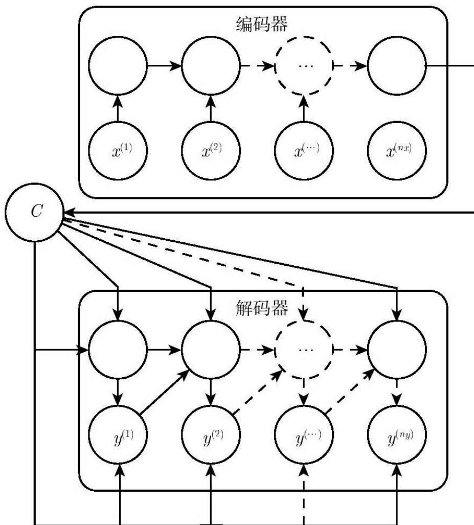
图10.12 在给定输入序列 (\mathbf{x}^{(1)}, \mathbf{x}^{(2)}, \dots, \mathbf{x}^{(n_x)}) 的情况下学习生成输出序列 (\mathbf{y}^{(1)}, \mathbf{y}^{(2)}, \dots, \mathbf{y}^{(n_y)}) 的编码器-解码器或序列到序列的RNN架构的示例。它由读取输入序
