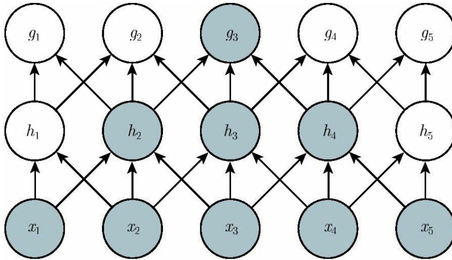
图9.4 处于卷积网络更深的层中的单元，它们的接受域要比处在浅层的单元的接受域更大。如果网络还包含类似步幅卷积（见图9.12）或者池化（第9.3节）之类的结构特征，这种效应会加强。这意味着在卷积网络中尽管直接连接都是很稀疏的，但处在更深的层中的单元可以间接地连接到全部或者大部分输入图像
