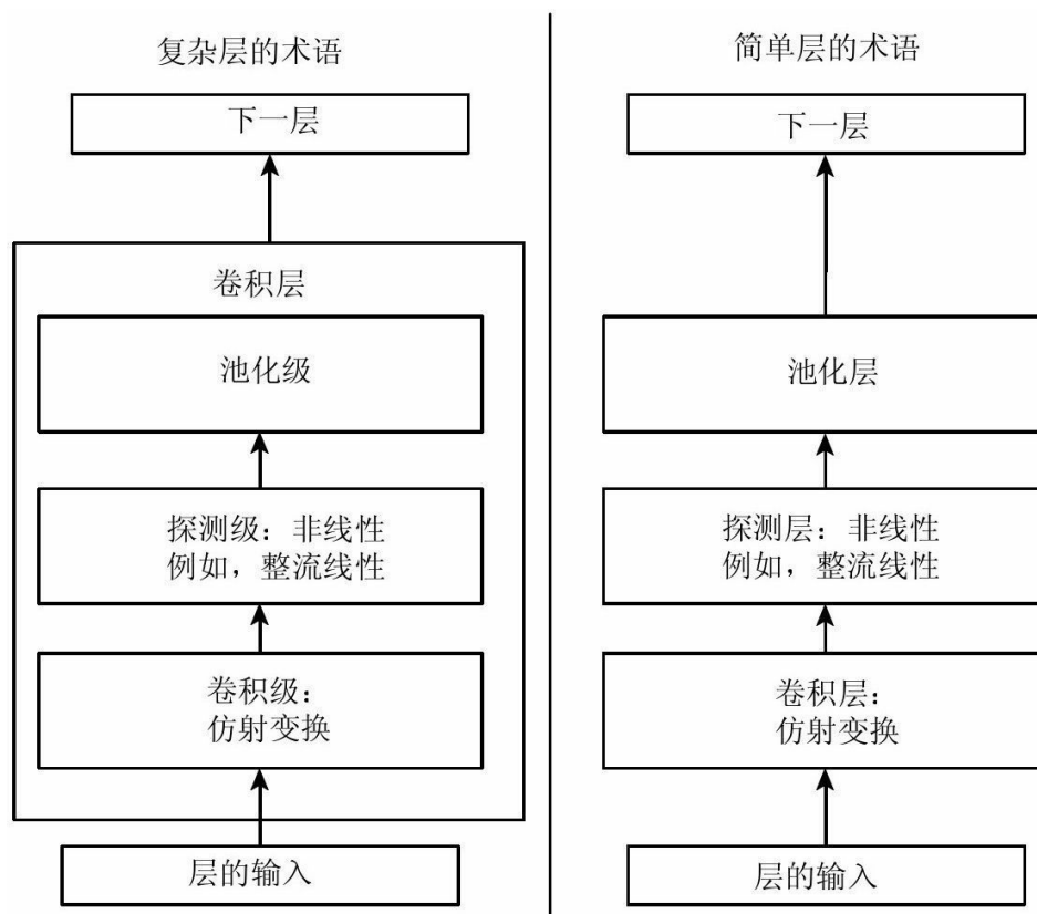
图9.7 一个典型卷积神经网络层的组件。有两组常用的术语用于描述这些层。（左）在这组术语中，卷积网络被视为少量相对复杂的层，每层具有许多“级”。在这组术语中，核张量与网络层之间存在一一对应关系。在本书中，我们通常使用这组术语。（右）在这组术语中，卷积网络被视为更多数量的简单层；每一个处理步骤都被认为是一个独立的层。这意味着不是每一“层”都有参数
