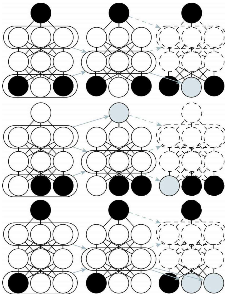
图20.5 深度玻尔兹曼机多预测训练过程的示意图。每一行指示相同训练步骤内小批量中的不同样本。每列表示均匀场推断过程中的时间步。对于每个样本，我们对数据变量的子集进行采样，作为推断过程的输入。这些变量以黑色阴影表示条件。然后我们运行均匀场推断过程，箭头指示过程中的哪些变量会影响其他变量。在实际应用中，我们将均匀场展开为几个步骤。在此示意图中，我们只展开为两个步骤。虚线箭头表示获得更多步骤需要如何展开该过程。未用作推断过程输入的数据变量成为目标，以灰色阴影表示。我们可以将每个样本的推断过程视为循环网络。为了使其在给定输入后能产生正确的目标，我们使用梯度下降和反向传播训练这些循环网络。这可以训练MP-DBM均匀场过程产生准确的估计。图改编自Goodfellow et al. (2013d)
