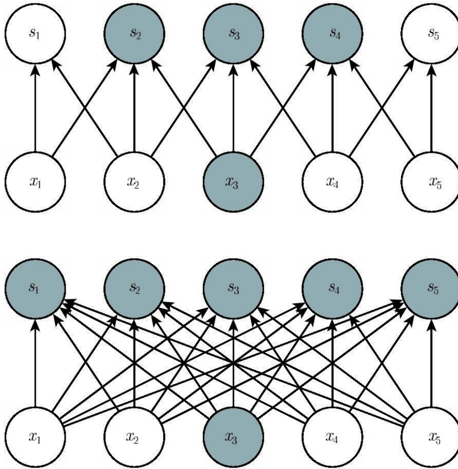
图9.2 稀疏连接，对每幅图从下往上看。我们强调了一个输入单元 x_3 以及在 s 中受该单元影响的输出单元。（上）当 s 是由核宽度为3的卷积产生时，只有3个输出受到 x 的影响。（下）当 s 是由矩阵乘法产生时，连接不再是稀疏的，所以所有的输出都会受到 x_3 的影响
