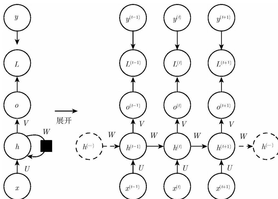
图10.3 计算循环网络（将 x 值的输入序列映射到输出值 o 的对应序列）训练损失的计算图。损失 L 衡量每个 o 与相应的训练目标 y 的距离。当使用softmax输出时，我们假设 o 是未归一化的数概率。损失 L 内部计算 \hat{y} = \text{softmax}(o) ，并将其与目标 y 比较。RNN输入到隐藏的连接由权重矩阵 U 参数化，隐藏到隐藏的循环连接由权重矩阵 W 参数化以及隐藏到输出的连接由权重矩阵 V 参数化。式（10.8）定义了该模型中的前向传播。（左）使用循环连接绘制的RNN和它的损失。（右）同一网络被视为展开的计算图，其中每个节点现在与一个特定的时间实例相关联
