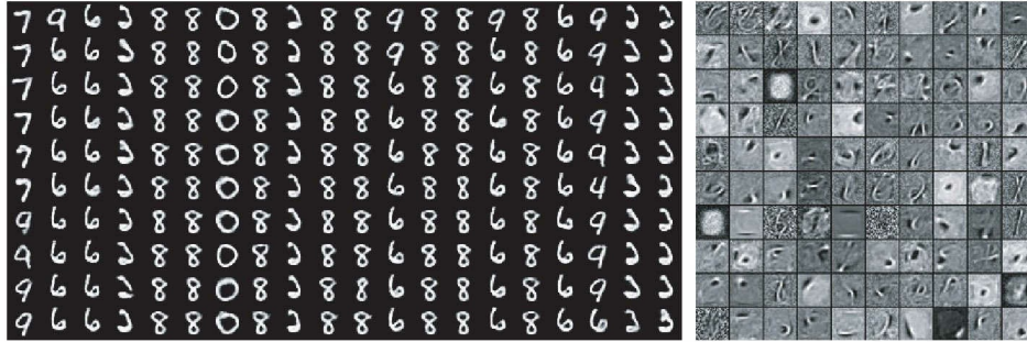
图16.15 训练好的RBM的样本及其权重。（左）用MNIST训练模型，然后用Gibbs采样进行采样。每一列是一个单独的Gibbs采样过程。每一行表示另一个1000步后Gibbs采样的输出。连续的样本之间彼此高度相关。（右）对应的权重向量。将本图结果与图13.2中描述的线性因子模型的样本和权重相比。由于RBM的先验 p(\mathbf{h}) 没有限制为因子，这里的样本表现得很好。采样时RBM能够学习到哪些特征需要一起出现。另一方面说，RBM后验 p(\mathbf{h} | \mathbf{v}) 是因子的，而稀疏编码的后验并不是，所以在特征提取上稀疏编码模型表现得更好。其他的模型可以使用非因子的 p(\mathbf{h}) 和非因子的 p(\mathbf{h} | \mathbf{v}) 。图片经LISA（2008）允许转载
