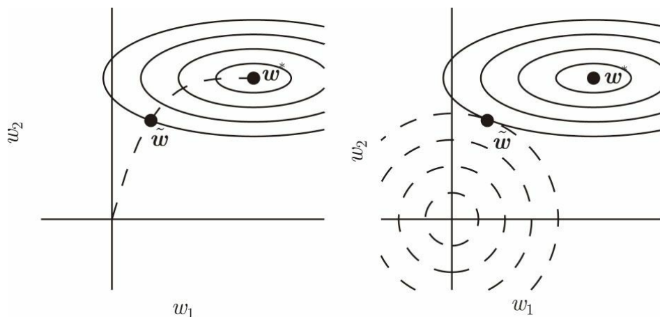
图7.4 提前终止效果的示意图。（左）实线轮廓线表示负对数似然的轮廓。虚线表示从原点开始的SGD所经过的轨迹。提前终止的轨迹在较早的点 \tilde{\mathbf{w}} 处停止，而不是停止在最小化代价的 \mathbf{w}^* 处。（右）为了对比，使用 L^2 正则化效果的示意图。虚线圆圈表示 L^2 惩罚的轮廓， L^2 惩罚使得总代价的最小值比非正则化代价的最小值更靠近原点
