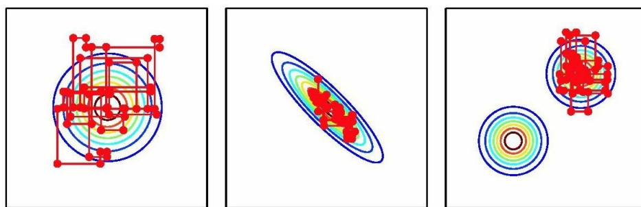
图17.1 对于三种分布使用Gibbs采样所产生的路径，所有的分布马尔可夫链初始值都设为峰值。（左）一个带有两个独立变量的多维正态分布。由于变量之间是相互独立的，Gibbs采样混合得很好。（中）变量之间存在高度相关性的一个多维正态分布。变量之间的相关性使得马尔可夫链很难混合。因为每一个变量的更新需要相对其他变量求条件分布，相关性减慢了马尔可夫链远离初始点的速度。（右）峰值之间间距很大且不在轴上对齐的混合高斯分布。Gibbs采样混合得很慢，因为每次更新仅仅一个变量很难跨越不同的峰值
