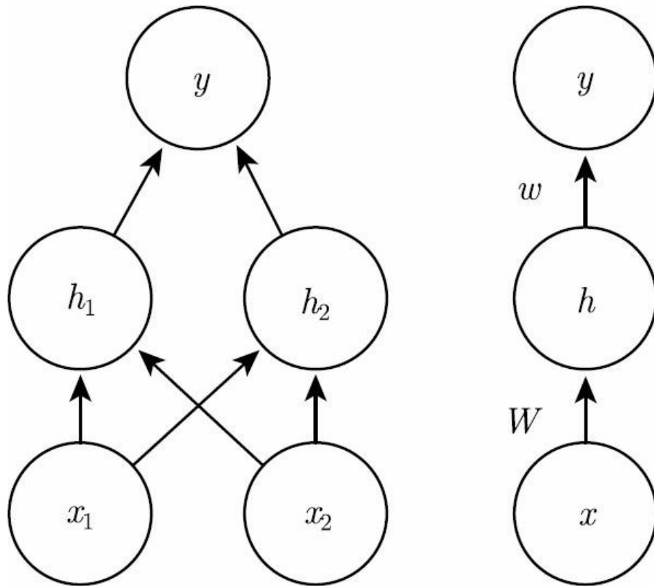
图6.2 使用两种不同样式绘制的前馈网络的示例。具体来说，这是我们来解决XOR问题的前馈网络。它有单个隐藏层，包含两个单元。（左）在这种样式中，我们将每个单元绘制为图中的一个节点。这种风格是清楚而明确的，但对于比这个例子更大的网络，它可能会消耗太多的空间。（右）在这种样式中，我们将表示每一层激活的整个向量绘制为图中的一个节点。这种样式更加紧凑。有时，我们对图中的边使用参数名进行注释，这些参数是用来描述两层之间的关系。这里，我们用矩阵 \mathbf{W} 描述从 \mathbf{x} 到 \mathbf{h} 的映射，用向量 \mathbf{w} 描述从 \mathbf{h} 到 y 的映射。当标这种图时，我们通常省略与每个层相关联的截距参数
