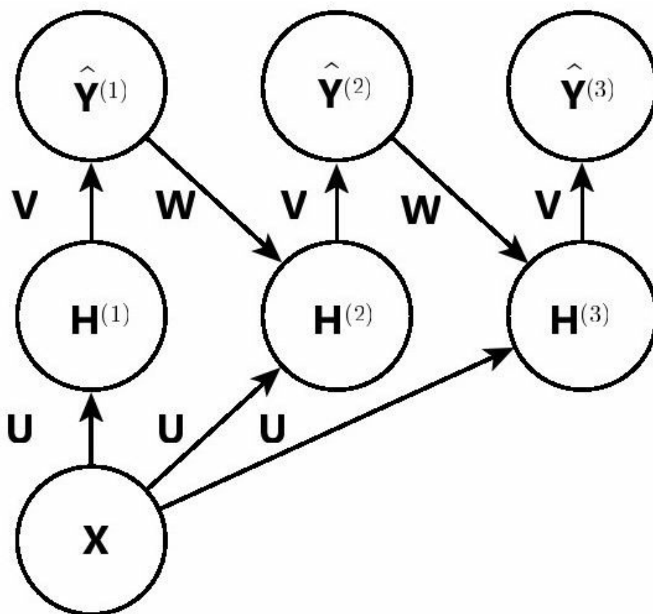
图9.17 用于像素标记的循环卷积网络的示例。输入是图像张量 X ，它的轴对应图像的行、列和通道（红、绿、蓝）。目标是输出标签 \hat{Y} ，它遵循每个像素的标签的概率分布。该张量的轴对应图像的行、列和不同类别。循环网络通过使用 \hat{Y} 的先前估计作为创建新估计的输入，来迭代地改善其估计，而不是单次输出 \hat{Y} 。每个更新的估计使用相同的参数，并且估计可以如我们所愿地被改善任意多次。每一步使用的卷积核张量 U ，是用来计算给定输入图像的隐藏表示的。核张量 V 用于产生给定隐藏值时标签的估计。除了第一步之外，核 W 都对 \hat{Y} 进行卷积来提供隐
