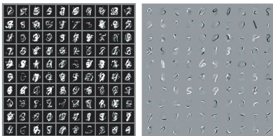
图13.2 尖峰和平板稀疏编码模型上在MNIST数据集训练的样例和权重。（左）这个模型中的样本和训练样本相差很大。第一眼看来，我们可能认为模型拟合得很差。（右）这个模型的权重向量已经学习到了如何表示笔迹，有时候还能写完整的数字。因此这个模型也学习到了有用的特征。问题在于特征的因子先验会导致特征子集合随机的组合。一些这样的子集能够合成可识别的MNIST集上的数字。这也促进了拥有更强大潜在编码分布的生成模型的发展。此图经
