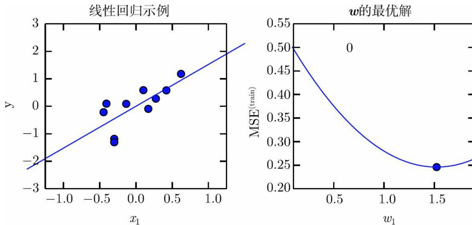
图5.1 一个线性回归问题，其中训练集包括10个数据点，每个数据点包含一个特征。因为只有一个特征，权重向量 \mathbf{w} 也只有一个要学习的参数 w_1 。（左）我们可以观察到线性回归学习 w_1 ，从而使得直线 y = w_1 x 能够尽量接近穿过所有的训练点。（右）标注的点表示由正规方程学习到的 w_1 的值，我们发现它可以最小化训练集上的均方误差
