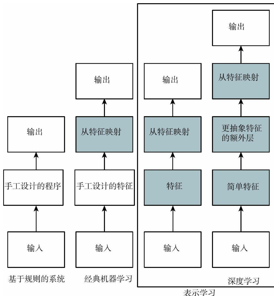
图1.5 流程图展示了AI系统的不同部分如何在不同的AI学科中彼此相关。阴影框表示能从数据中学习的组件
