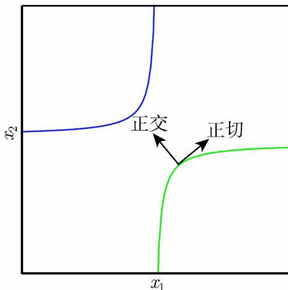
图7.9 正切传播算法（Simard et al. ，1992）和流形正切分类器主要思想的示意图（Rifai et al. ，2011c），它们都正则化分类器的输出函数 f(\mathbf{x}) 。每条曲线表示不同类别的流形，这里表示嵌入二维空间中的一维流形。在一条曲线上，我们选择单个点并绘制一个与类别流形（平行并接触流形）相切的向量以及与类别流形（与流形正交）垂直的向量。在多维情况下，可以存在许多切线方向和法线方向。我们希望分类函数在垂直于流形方向上快速改变，并且在类别流形的方向上保持不变。正切传播和流形正切分类器都会正则化 f(\mathbf{x}) ，使其不随 \mathbf{x} 沿流形的移动而剧烈变化。正切传播需要用户手动指定正切方向的计算函数（例如指定小平移后的图像保留在相同类别的流形中），而流形正切分类器通过训练自编码器拟合训练数据来估计流形的正切方向。我们将在第14章中讨论使用自编码器来估计流形
