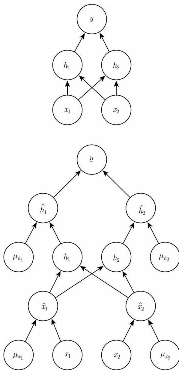
图7.7 在使用Dropout的前馈网络中前向传播的示例。（顶部）在此示例中，我们使用具有两个输入单元，具有两个隐藏单元的隐藏层以及一个输出单元的前馈网络。（底部）为了执行具有Dropout的前向传播，我们随机地对向量 \mu 进行采样，其中网络中的每个输入或隐藏单元对应一项。 \mu 中的每项都是二值的且独立于其他项采样。超参数的采样概率为1，隐藏层的采样概率通常为0.5，输入的采样概率通常为0.8。网络中的每个单元乘以相应的掩码，然后正常地继续沿着网络的其余部分前向传播。这相当于从图7.6中随机选择一个子网络并沿着前向传播
