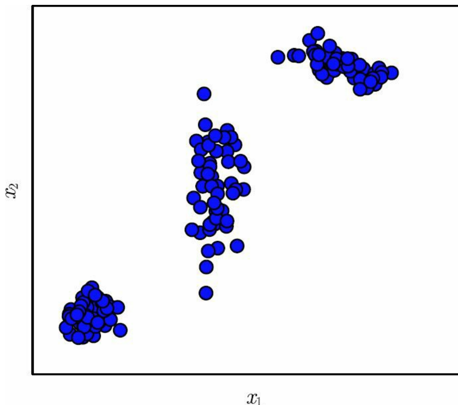
图3.2 来自高斯混合模型的样本。在这个示例中，有3个组件。从左到右，第1个组件具有各向
