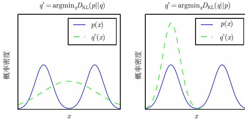
图3.6 KL散度是不对称的。假设我们有一个分布 P(x) ，并且希望用另一个分布 q(x) 来近似它。我们可以选择最小化 D_{KL}(p||q) 或最小化 D_{KL}(q||p) 。为了说明每种选择的效果，我们令 p 是两个高斯分布的混合，令 q 为单个高斯分布。选择使用KL散度的哪个方向是取决于问题的。一些应用需要这个近似分布 q 在真实分布 p 放置高概率的所有地方都放置高概率，而其他应用需要这个近似分布 q 在真实分布 p 放置低概率的所有地方都很少放置高概率。KL散度方向的选择反映了对于每种应用，优先考虑哪一种选择。（左）最小化 D_{KL}(p||q) 的效果。在这种情况下，我们选择一个 q ，使得它在 p 具有高概率的地方具有高概率。当 p 具有多个峰时， q 选择将这些峰模糊到一起，以便将高概率质量放到所有峰上。（右）最小化 D_{KL}(q||p) 的效果。在这种情况下，我们选择一个 q ，使得它在 p 具有低概率的地方具有低概率。当 p 具有多个峰并且这些峰间隔很宽时，如该图所示，最小化KL散度会选择单个峰，以避免将概率质量放置在 p 的多个峰之间的低概率区域中。这里，我们说明当 q 被选择成强调左边峰时的结果。我们也可以通过选择右边峰来得到KL散度相同的值。如果这些峰没有被足够强的低概率区域分离，那么KL散度的这个方向仍然可能选择模糊这些峰
