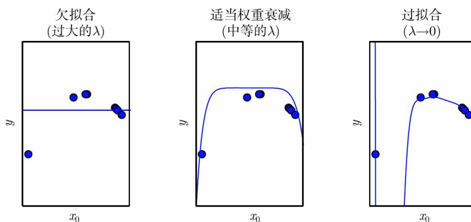
图5.5 我们使用高阶多项式回归模型来拟合图5.2中的训练样本。真实函数是二次的，但是在这里只使用9阶多项式。我们通过改变权重衰减的量来避免高阶模型的过拟合问题。（左）当 \lambda 非常大时，我们可以强迫模型学习到一个没有斜率的函数。由于它只能表示一个常数函数，所以会导致欠拟合。（中）取一个适当的 \lambda 时，学习算法能够用一个正常的形状来恢复曲率。即使模型能够用更复杂的形状来表示函数，权重衰减也鼓励用一个带有更小参数的更简单的模型来描述它。（右）当权重衰减趋近于0（即使用Moore-Penrose伪逆来解这个带有最小正则化的欠定
