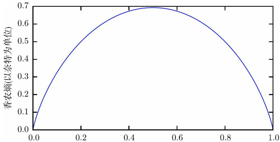
图3.5 二值随机变量的香农熵。该图说明了更接近确定性的分布是如何具有较低的香农熵，而更接近均匀分布的分布是如何具有较高的香农熵。水平轴是 p ，表示二值随机变量等于1的概率。熵由 (p-1)\log(1-p)-p \log p 给出。当 p 接近0时，分布几乎是确定的，因为随机变量几乎总是0。当 p 接近1时，分布也几乎是确定的，因为随机变量几乎总是1。当 p=0.5 时，熵是最大的，因为分布在两个结果（0和1）上是均匀的
