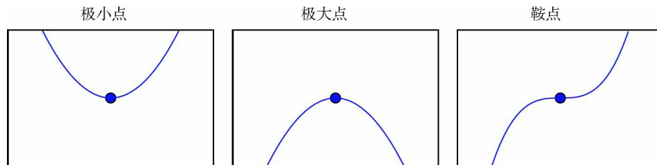
图4.2 临界点的类型。一维情况下，3种临界点的示例。临界点是斜率为零的点。这样的点可以是：局部极小点（local minimum），其值低于相邻点；局部极大点（local maximum），其值高于相邻点；鞍点，同时存在更高和更低的相邻点
