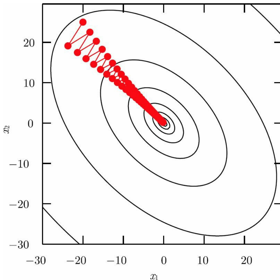
图4.6 梯度下降无法利用包含在Hessian矩阵中的曲率信息。这里我们使用梯度下降来最小化Hessian矩阵条件数为5的二次函数 f(\mathbf{x}) 。这意味着最大曲率方向具有比最小曲率方向多5倍的曲率。在这种情况下，最大曲率在 [1, 1]^T 方向上，最小曲率在 [1, -1]^T 方向上。红线表示梯度下降的路径。这个非常细长的二次函数类似一个长峡谷。梯度下降把时间浪费于在峡谷壁反复下降，因为它们是最陡峭的特征。由于步长有点大，有超过函数底部的趋势，因此需要在下一次迭代时在对面的峡谷壁下降。与指向该方向的特征向量对应的Hessian的大正特征值表示该方向上的导数快速增加，因此基于Hessian的优化算法可以预测，在此情况下最陡峭方向实际上不是有前途的搜索方向
