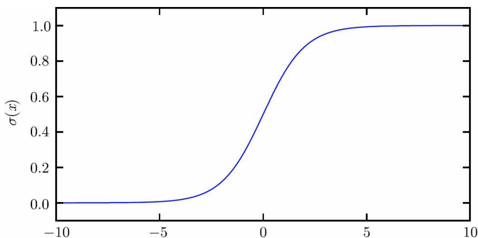
图3.3 logistic sigmoid函数
