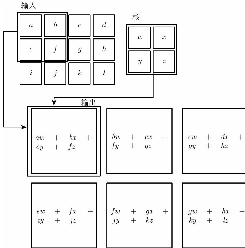
图9.1 一个二维卷积的例子（没有对核进行翻转）。我们限制只对核完全处在图像中的位置进行输出，在一些上下文中称为“有效”卷积。我们用画有箭头的盒子来说明输出张量的左上角元素是如何通过对输入张量相应的左上角区域应用核进行卷积得到的
