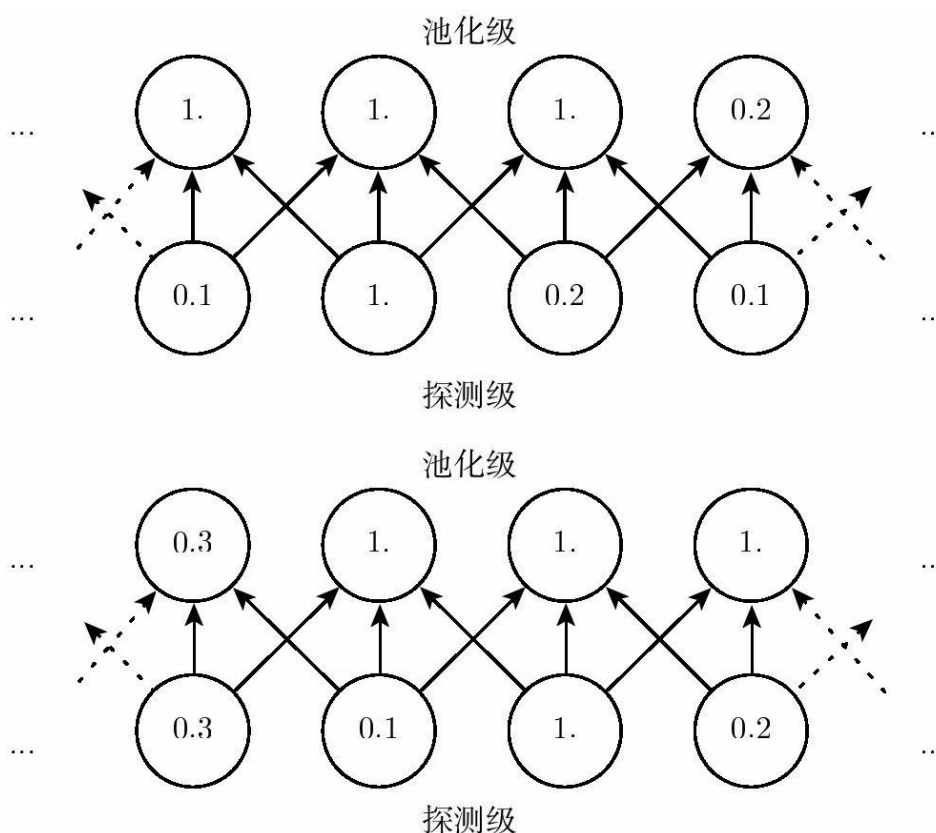
图9.8 最大池化引入了不变性。（上）卷积层中间输出的视图。下面一行显示非线性的输出。上面一行显示最大池化的输出，每个池的宽度为三个像素并且池化区域的步幅为一个像素。（下）相同网络的视图，不过对输入右移了一个像素。下面一行的所有值都发生了改变，但上面一行只有一半的值发生了改变，这是因为最大池化单元只对周围的最大值比较敏感，而不是对精确的位置
