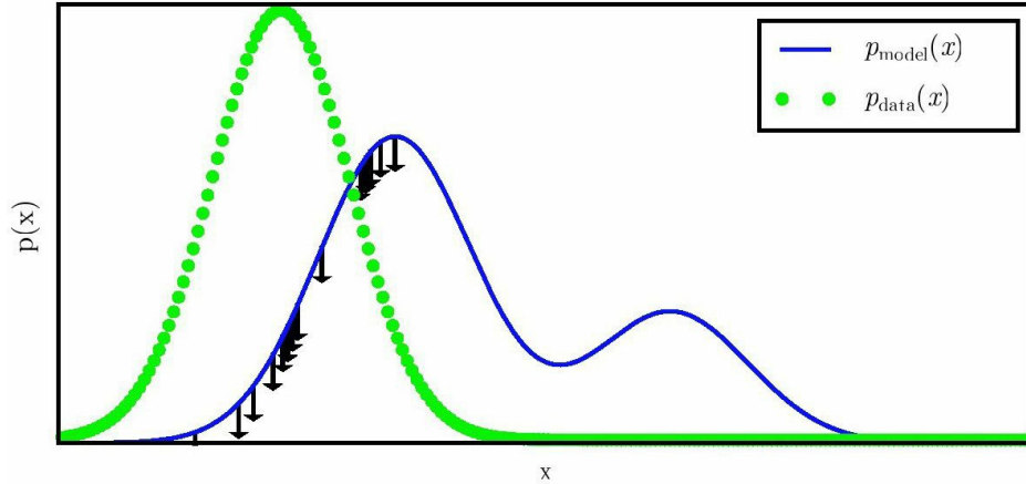
图18.2 一个虚假模态。说明对比散度（算法18.2）的负相为何无法抑制虚假模态的例子。一个虚假模态指的是一个在模型分布中出现数据分布中却不存在的模式。由于对比散度从数据点中初始化它的马尔可夫链然后仅仅运行了几步马尔可夫链，不太可能到达模型中离数据点较远的模式。这意味着从模型中采样时，我们有时候会得到一些与数据并不相似的样本。这也意味着由于在这些模式上浪费了一些概率质量，模型很难把较高的概率质量集中于正确的模式上。出于可视化的目的，这个图使用了某种程度上更加简单的距离的概念——在 \mathbb{R} 的数轴上虚假模式与正确的模式有很大的距离。这对应着基于局部移动 \mathbb{R} 上的单个变量 x 的马尔可夫链。对于大部分深度概率模型来说，马尔可夫链是基于Gibbs采样的，并且对于单个变量产生非局部的移动但是无法同时移动所有的变量。对于这些问题来说，考虑编辑距离比欧式距离通常更好。然而，高维空间的编辑距离很难在二维空间作图展示
